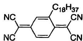
C 18 TCNQ
