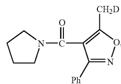
1-[[5-(methyl-d)-3-phenyl-4-isoxazolyl]carbonyl]-pyrrolidine
