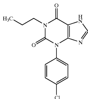
Arofylline (LAS-31025)
