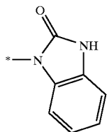
1H-benzimidazol-2-on-3-yl
