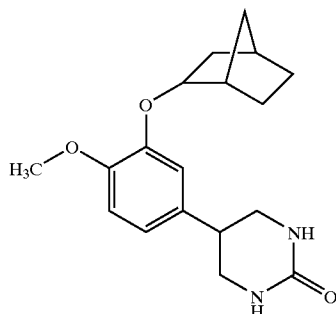
Atizoram (CP-80,633)
