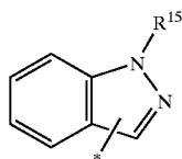
1H-indazolyl
