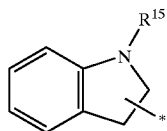
indoliny
