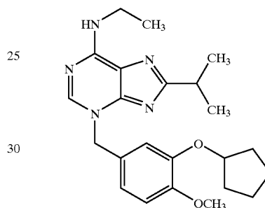
V-11294A
