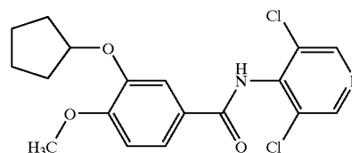
Piclamilast (RP-73,401)
