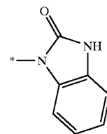
1H-benzimidazol-2- on-3-yl
