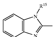
benzimidazolyl
