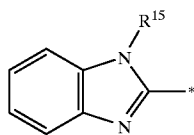
benzoimidazolyl
