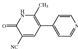
Milrinone
