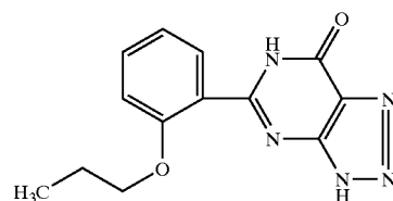
Zaprinast
