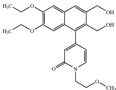
T-440
