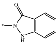
1H-indazol-3-on-2-yl
