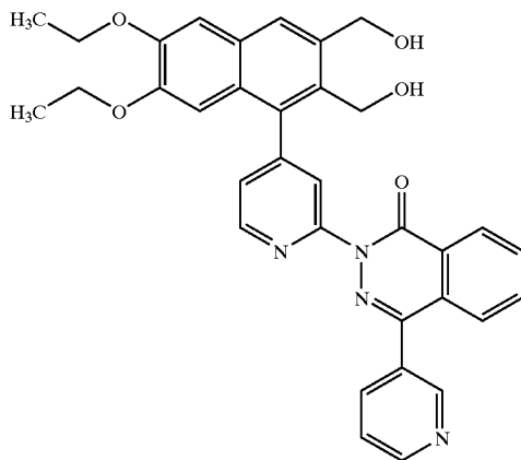
T-2585
