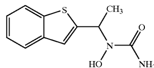
ZYFLO® Zileuton
