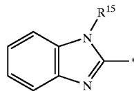
benzimidazolyl
