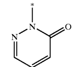
pyridazin-3-on-2-yl
