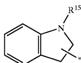
indoliny
