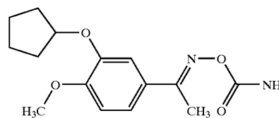
Filaminast (WAY-PDA-641)
