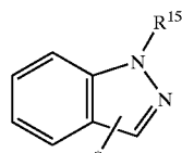
1H-indazolyl
