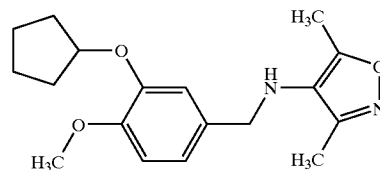
RPR-132294
