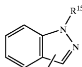
1H-indazolyl
