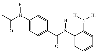
CI-994
