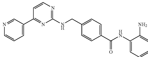
N-(2-Aminophenyl)-4-[[4-(pyridin-3-yl)pyrimidin-2-yl]amino]methyl]benzamide
