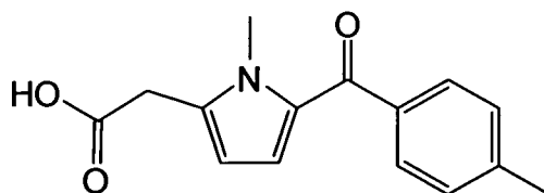
Tolmetin
