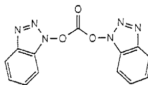
Di(1-benzotriazolyl) carbonate
