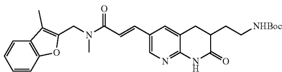
Tert-butyl (E)-(2-(6-(3-(methyl((3-methylbenzofuran-2-yl)methyl)amino)-3-oxoprop-1-en-1-yl)-2-oxo-1,2,3,4-tetrahydro-1,8-naphthyridin-3-yl)ethyl)carbamate (E-16)
