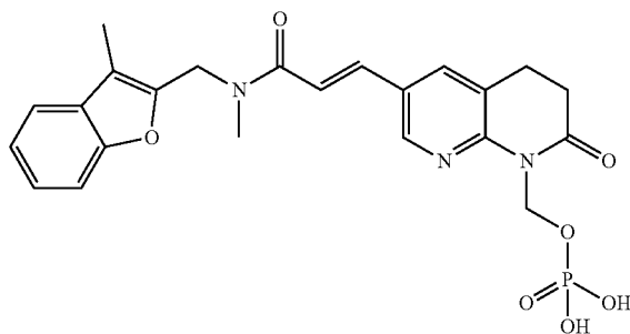
Afabacin (Debio 1450)
