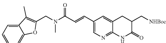
Tert-butyl(E)-((6-(3-(methyl((3-methylbenzofuran-2-yl)methyl)amino)-3-oxoprop-1-en-1-yl)-2-oxo-1,2,3,4-tetrahydro-1,8-naphthyridin-3-yl)methyl)carbamate (E-12)
