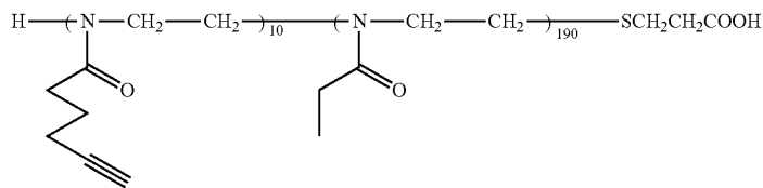
H-[(Plyn) 10 (EOZ) 190 ]-COOH 20K
