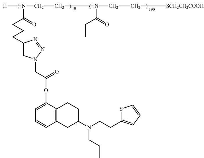
H-[(Acetyl-Rotigotine) 10 (EOZ) 190 ]-COOH 20K
