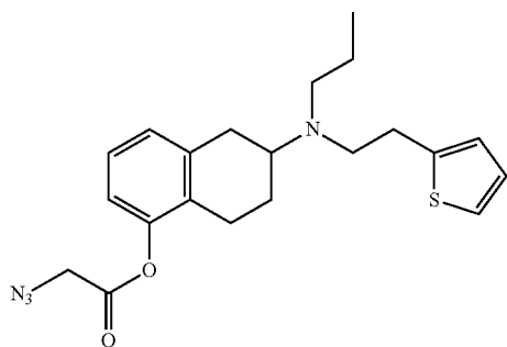
Azidoacetyl-Rotigotine
