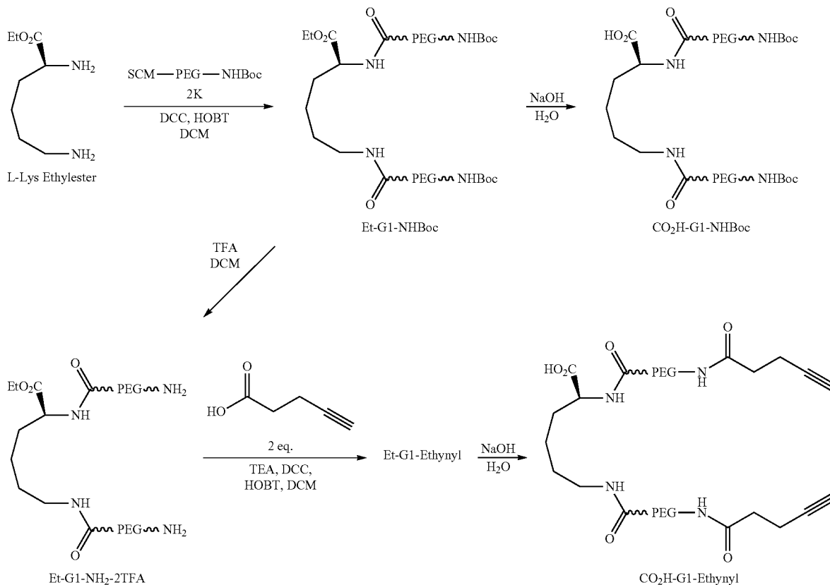
Et-G1-NHBoc
