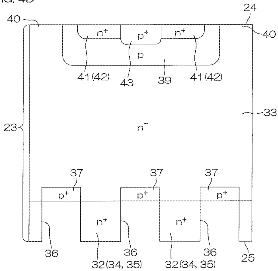
FIG. 4D
