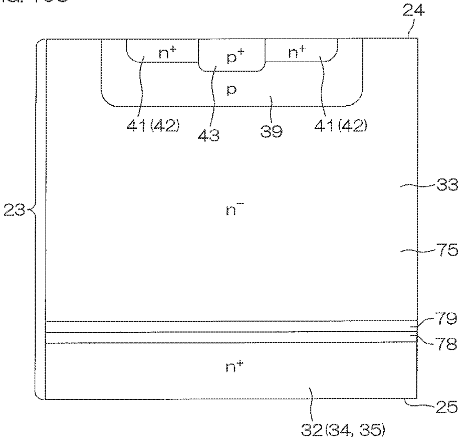
FIG. 10C
