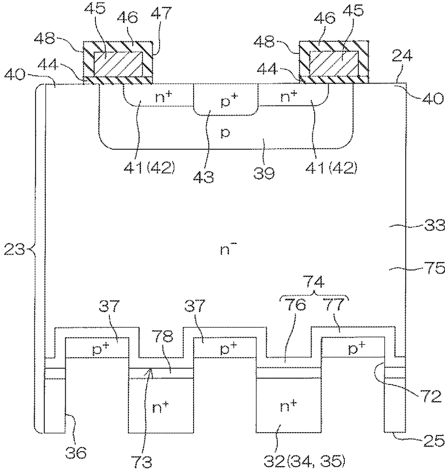
FIG. 10G
