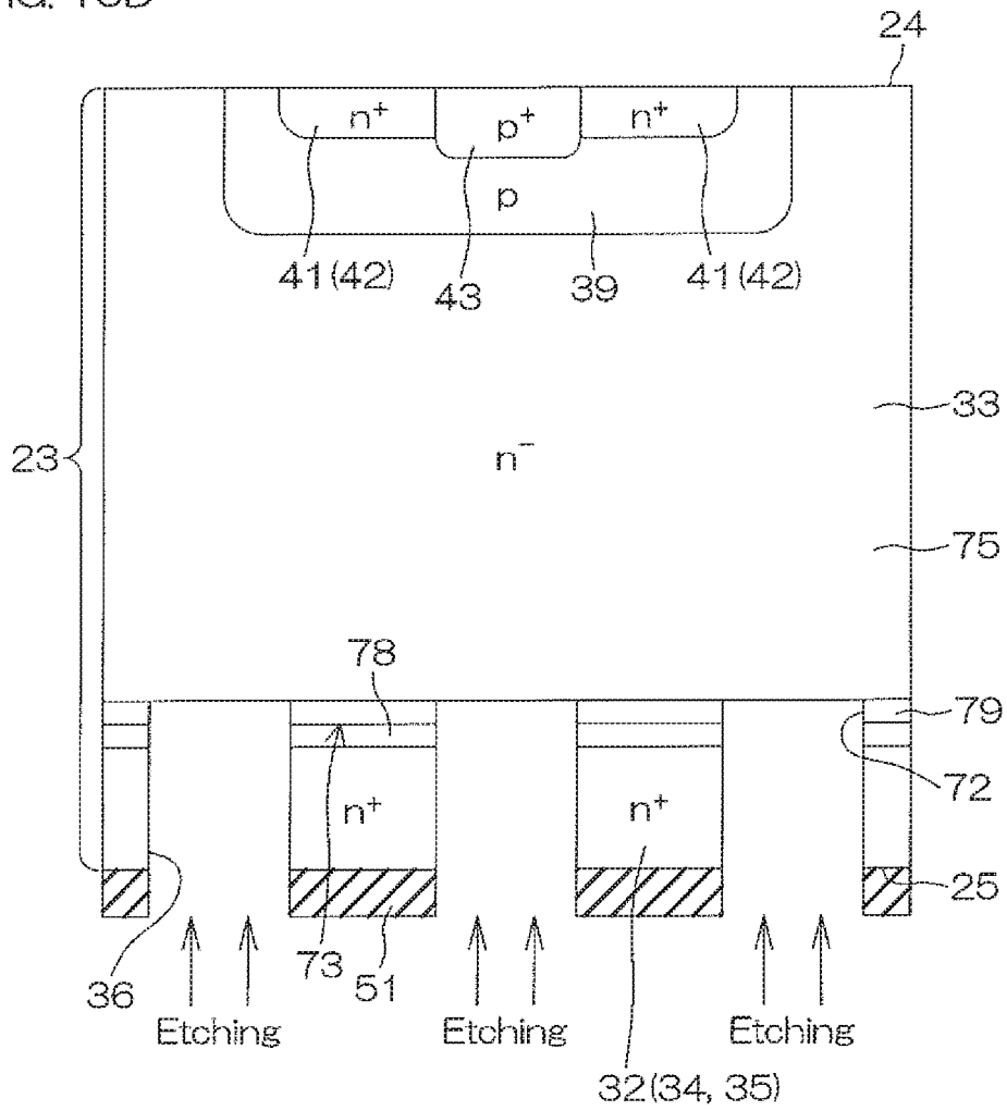
FIG. 10D
