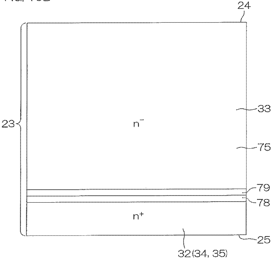
FIG. 10B
