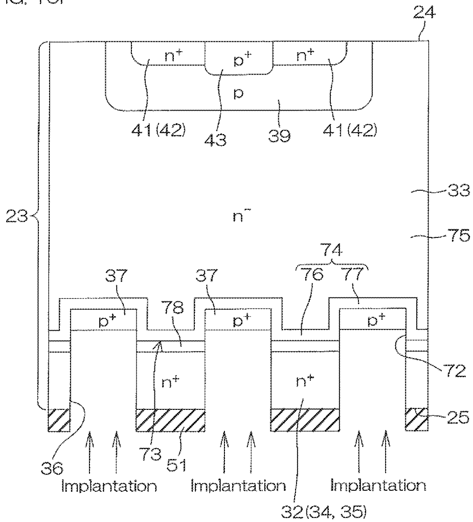
FIG. 10F
