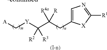
(I-n)
