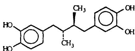
Nordihydroguaiaretic Acid
