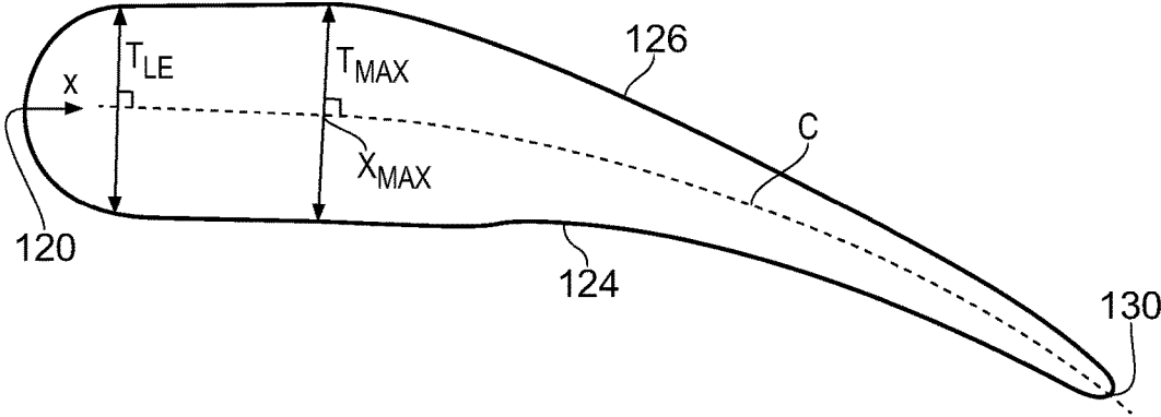
SECTION A-A FIG. 4
