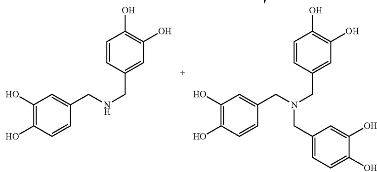
DC-0075
