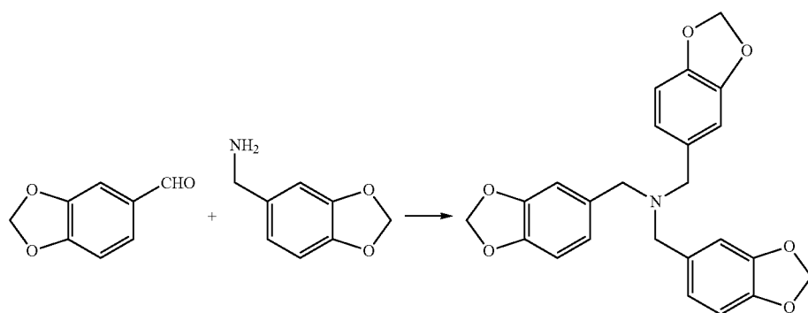
DC-0075B
