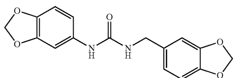
1-(3,4-methylenedioxyphenyl)-3-(3,4-methylenedioxybenzyl) urea
