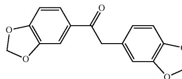
bis(3,4-methylenedioxy)desoxybenzoin
