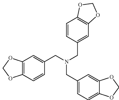
tris-(3,4-methylenedioxybenzyl)-amine
