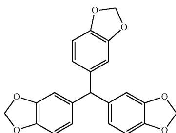
Tris-(3,4-methylenedioxyphenyl)methane
