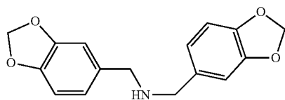
bis-(3,4-methylenedioxybenzyl)-amine
