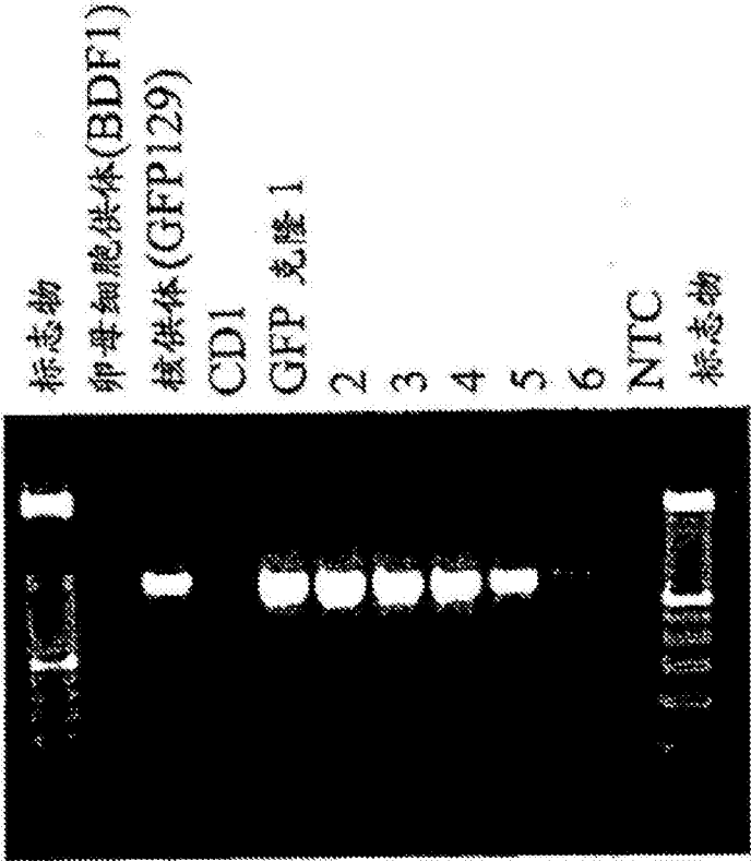
基因组 DNA
