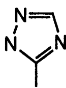
Triazoles
