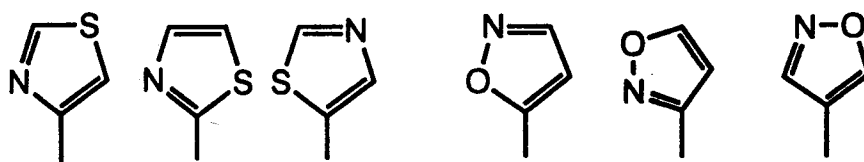
Isoxazoles
