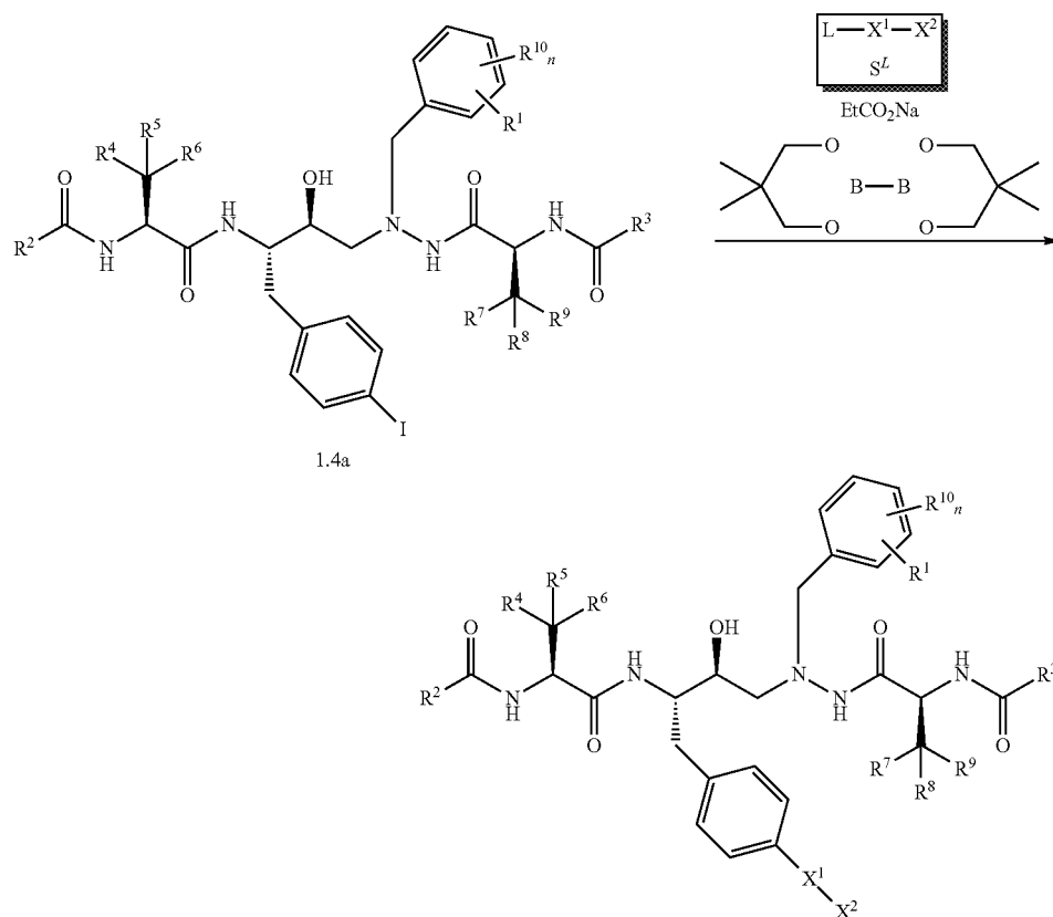
SCHEME 1.4
