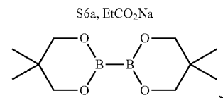
S6a, EtCO 2 Na
