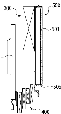
(B) A—A断面图
