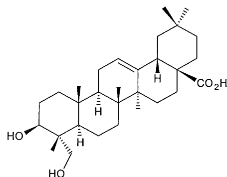
Hederagenin
