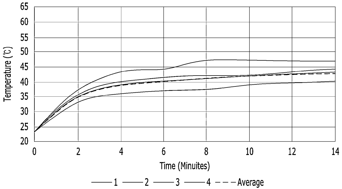
FIG. 16D
