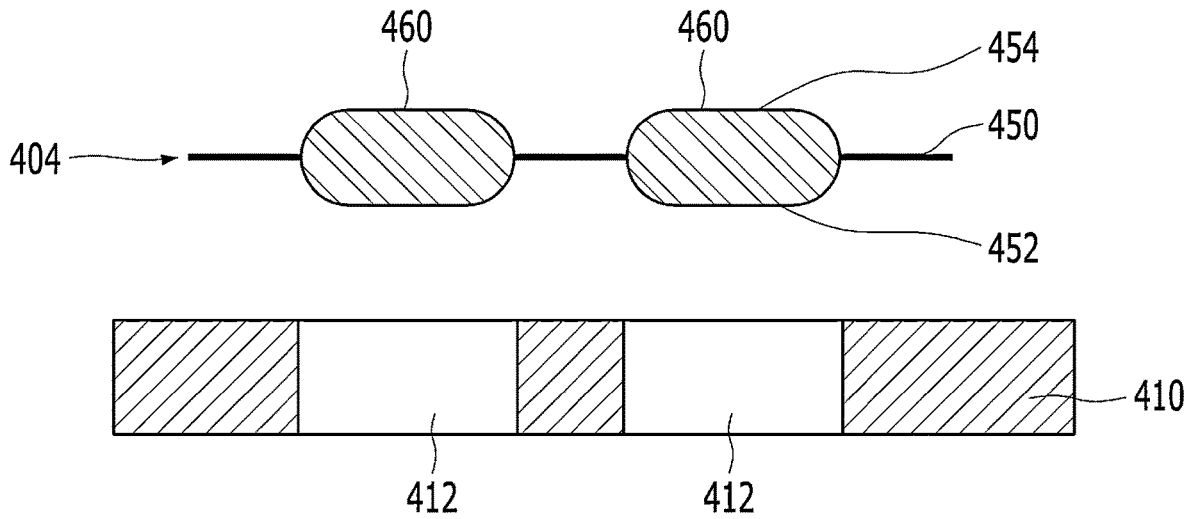
FIG. 4J
