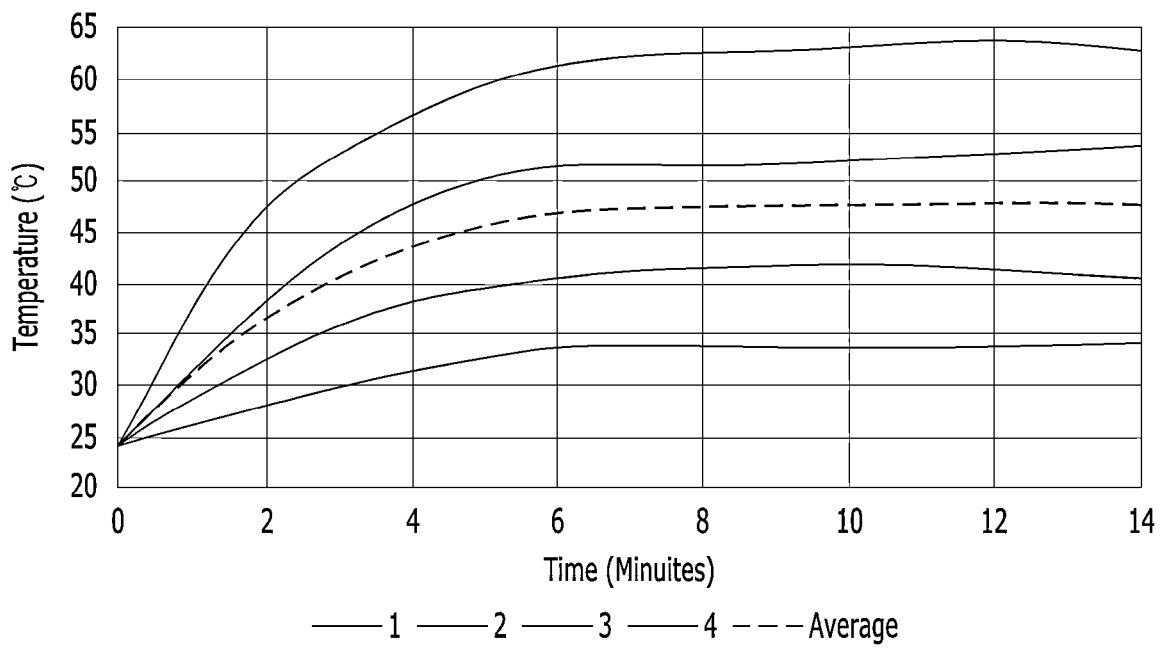
FIG. 16C
