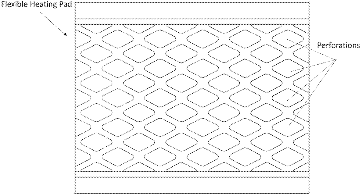
FIG. 17A
