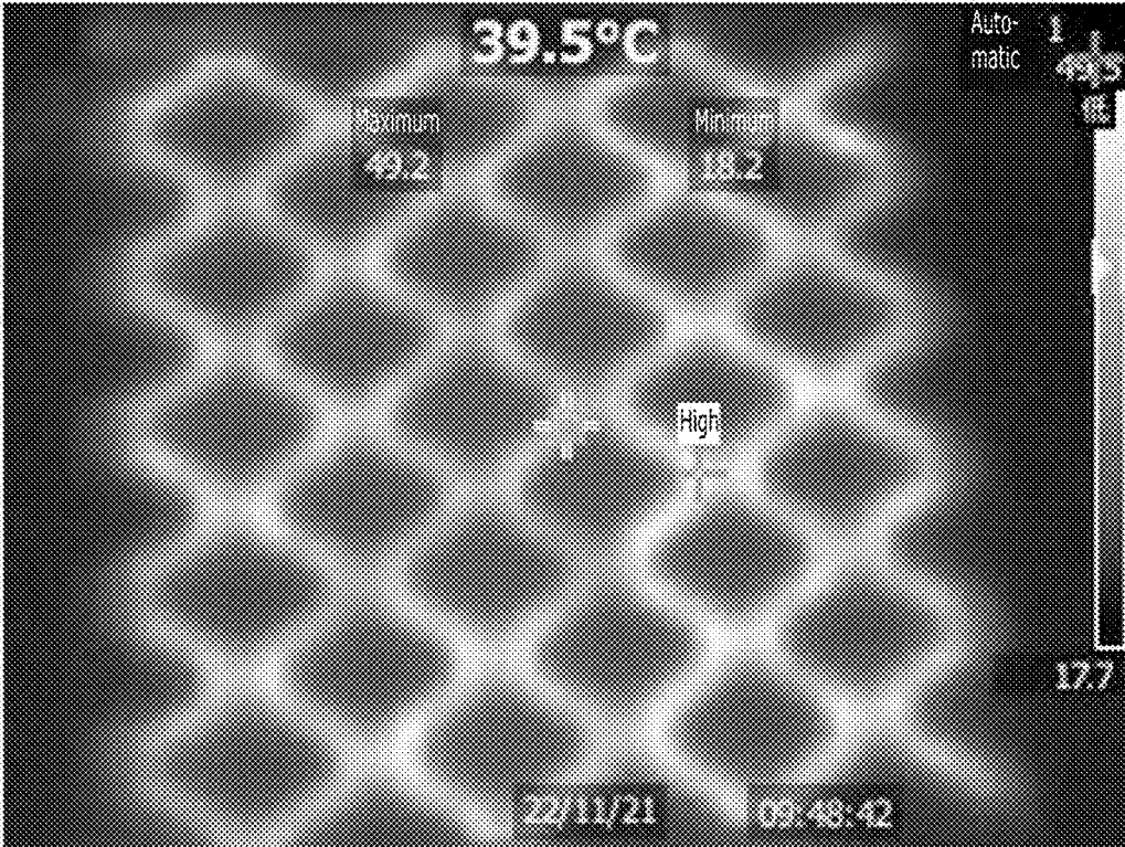
FIG. 17B
