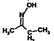
MEK oxime
