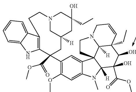
Des-acetyl Vinblastine
