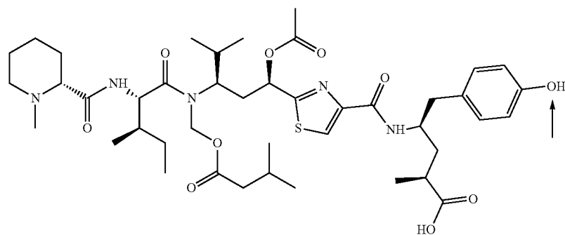
Tubulysin A
