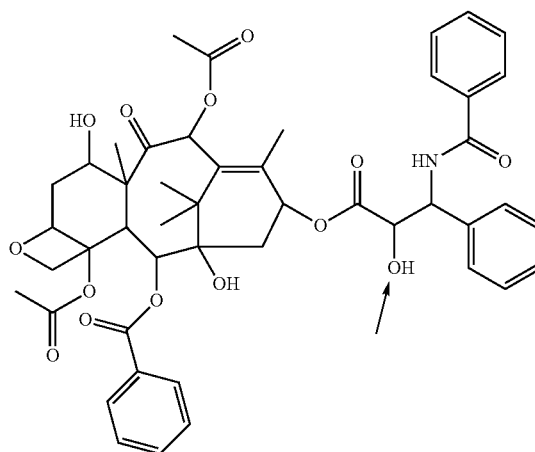
Paclitaxel
