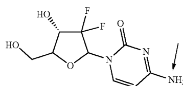
Gemcitabine
