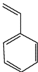
STYRENE
