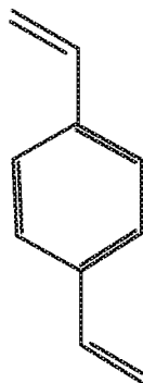
DIVINYLBENZENE
