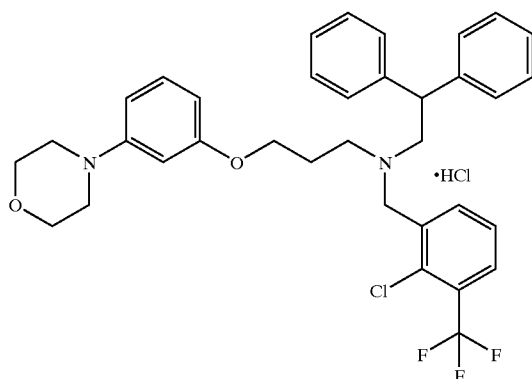
a) (2,2-Diphenylethyl)(2-chloro-3-trifluoromethyl-benzyl)amine
