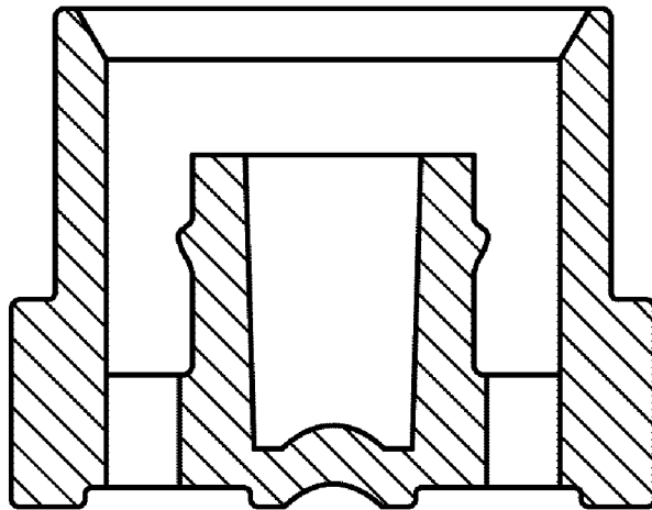
【A-A線剖面圖】
