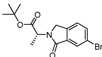
tert-butyl (R)-2-(6-bromo-1-oxoisindolin-2-yl)propanoate
