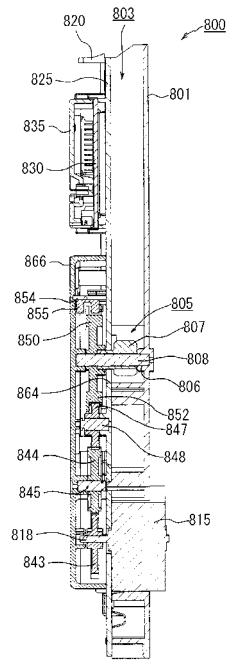
A-A断面図
