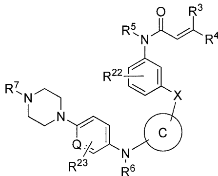
Formula Ic
