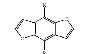
benzodifuran
