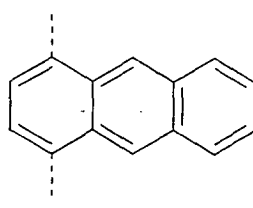
Formel (LXIV)
