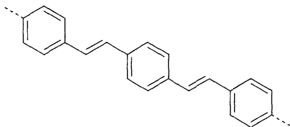
Formel (LXVIII)
