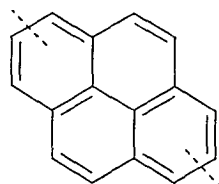
Formel (LXI)
