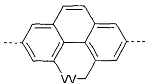
Formel (LXIX)
