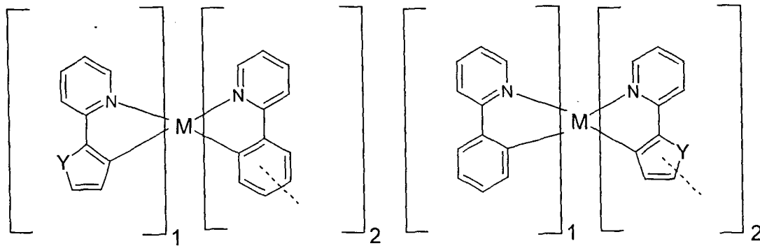
Formel (LII)
