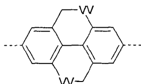
Formel (LXXIII)
