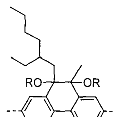
Formel (CI)
