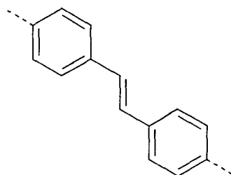
Formel (LXVII)
