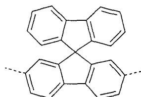
Formel (LXXIV)
