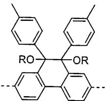
Formel (LXXXIV)
