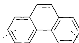
Formel (LXV)
