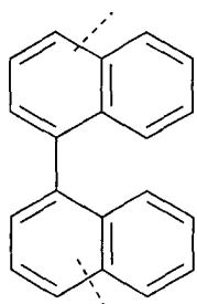
Formel (LXVI)
