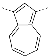
Formel (XIV)
