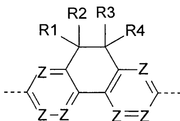
FORMEL (Ia)
