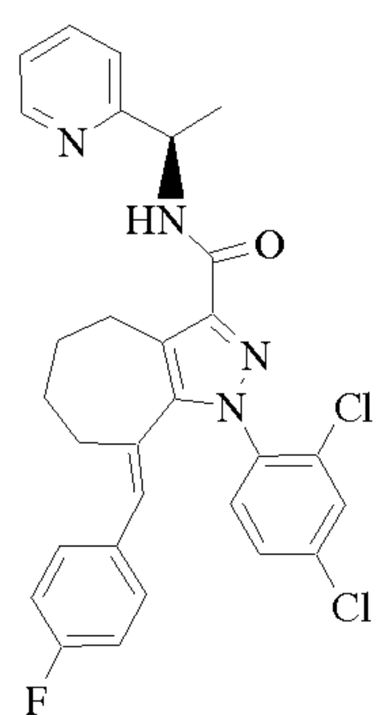
Cpd 225
