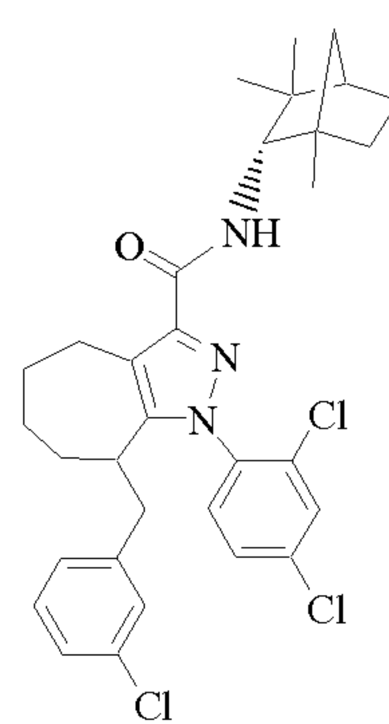
Cpd 15
