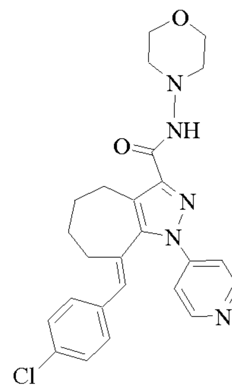
Cpd 179
