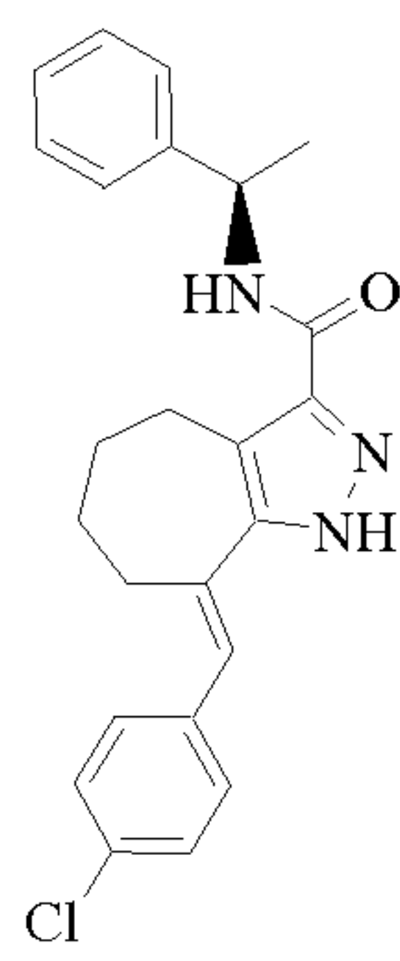
Cpd 142
