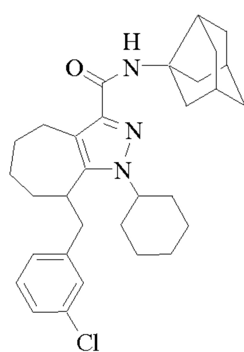
Cpd 5
