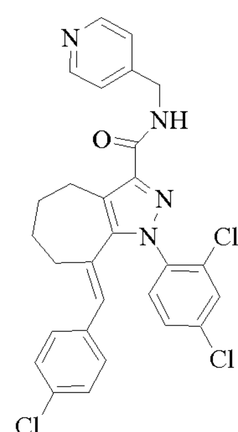
Cpd 152
