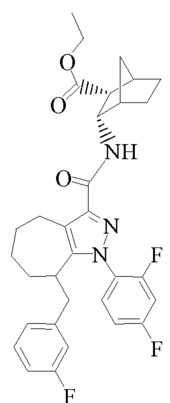
Cpd 111
