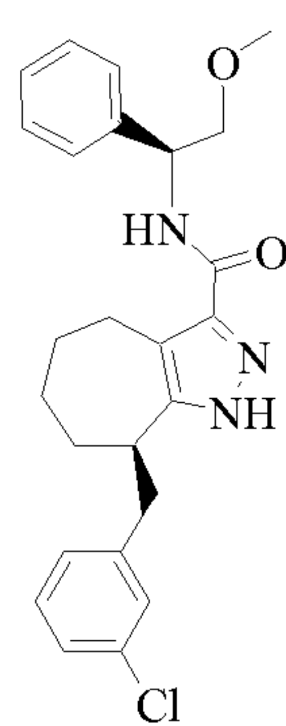
Cpd 251
