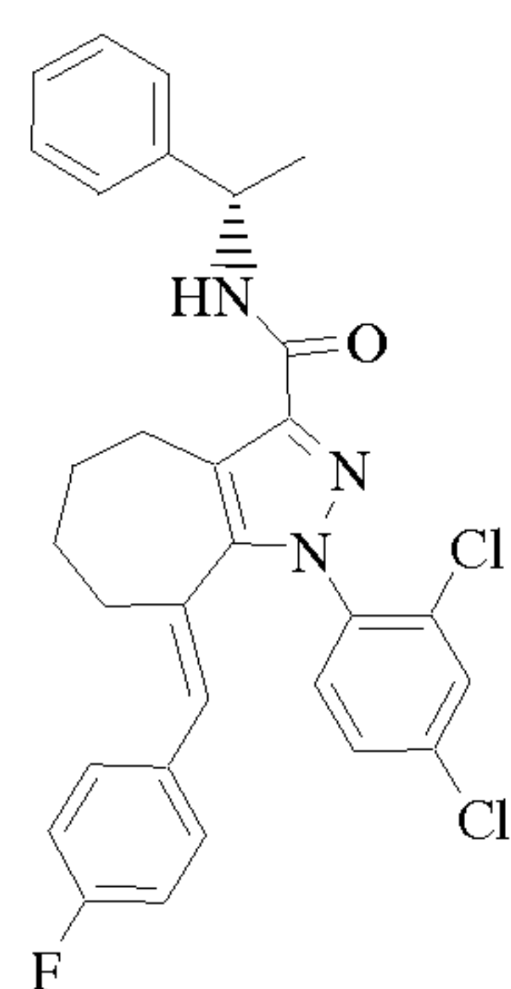
Cpd 149
