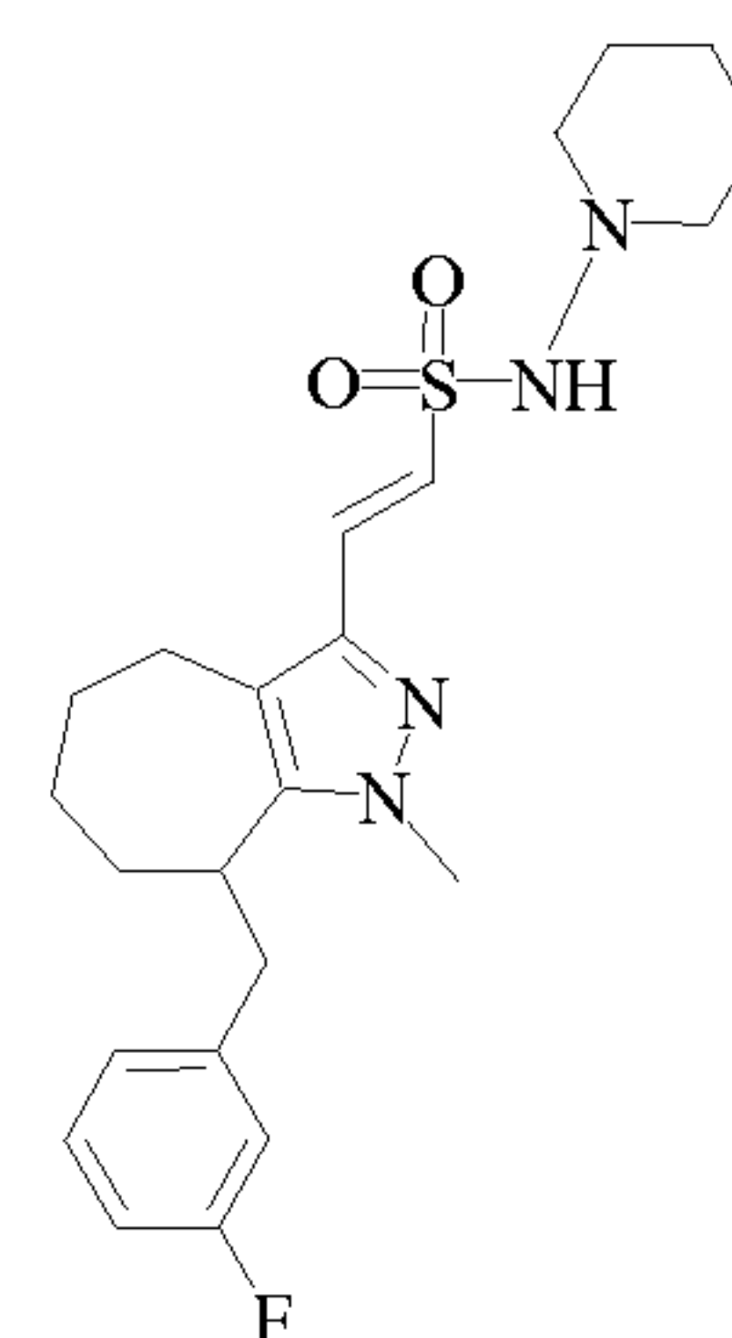
Cpd 120
