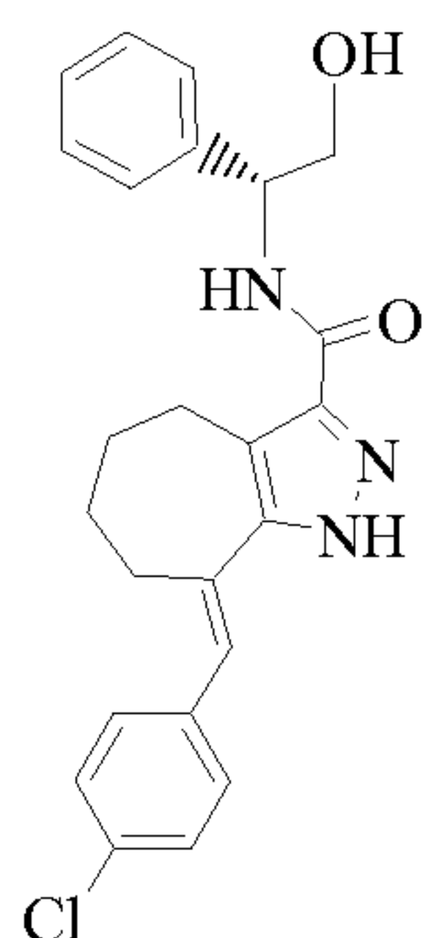
Cpd 230
