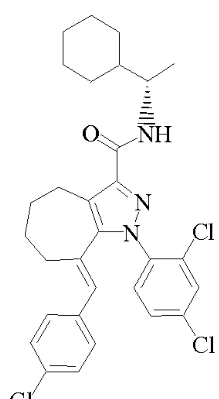
Cpd 138
