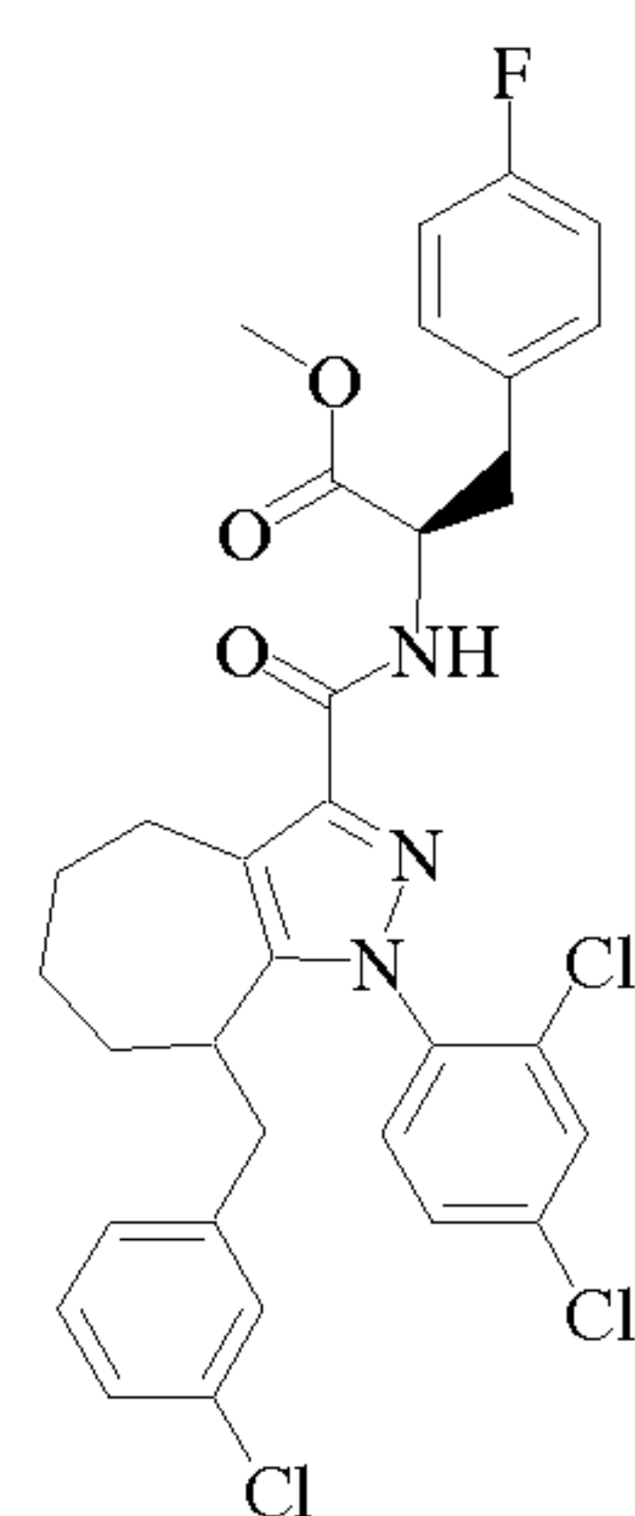
Cpd 103
