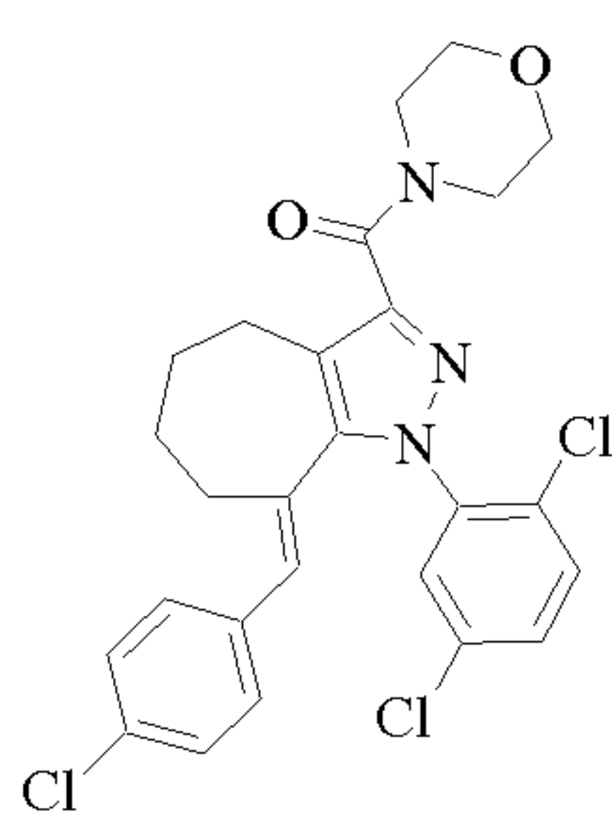
Cpd 197
