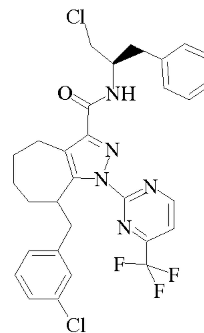
Cpd 183
