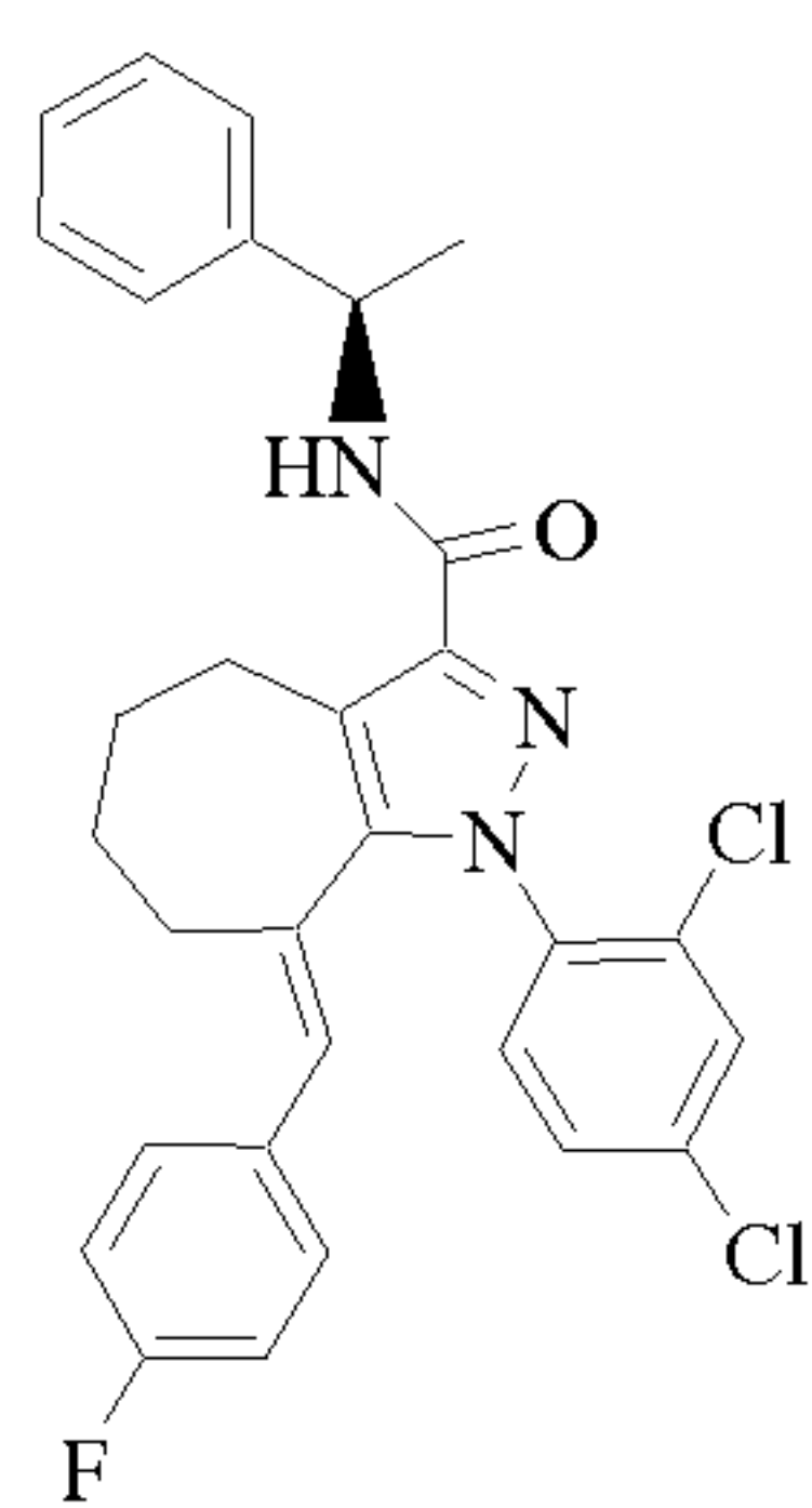
Cpd 146
