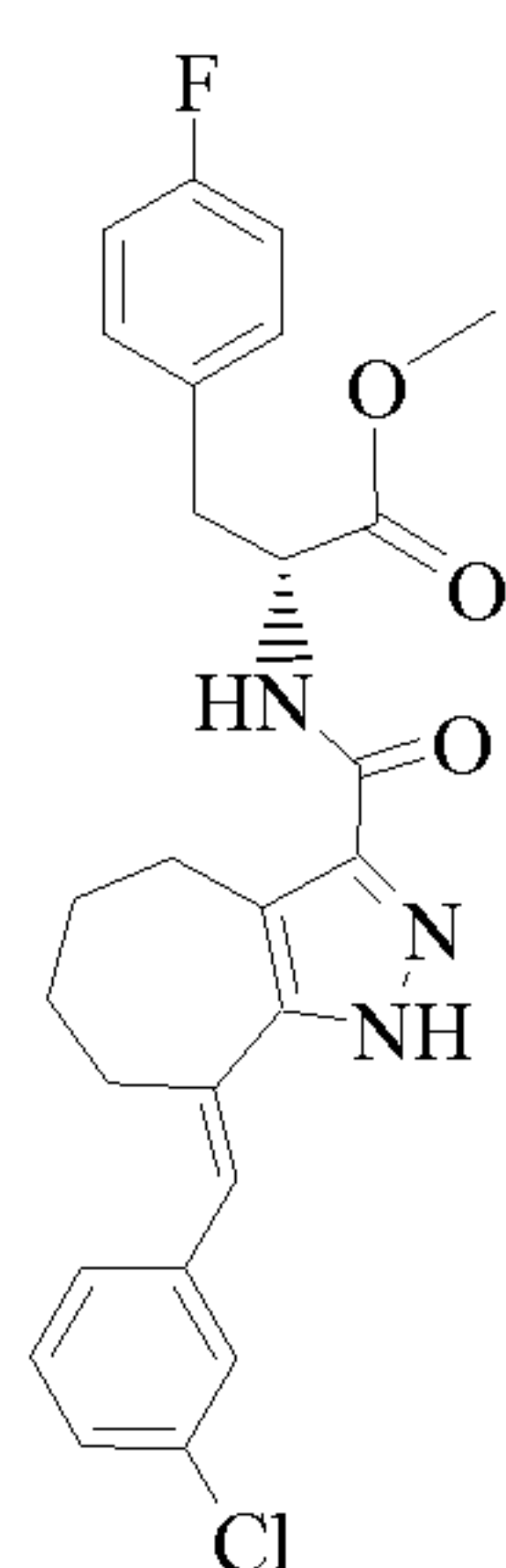
Cpd 245
