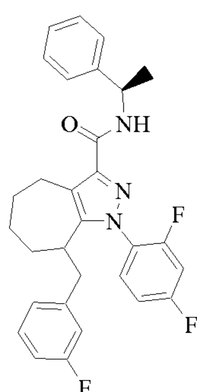
Cpd 173
