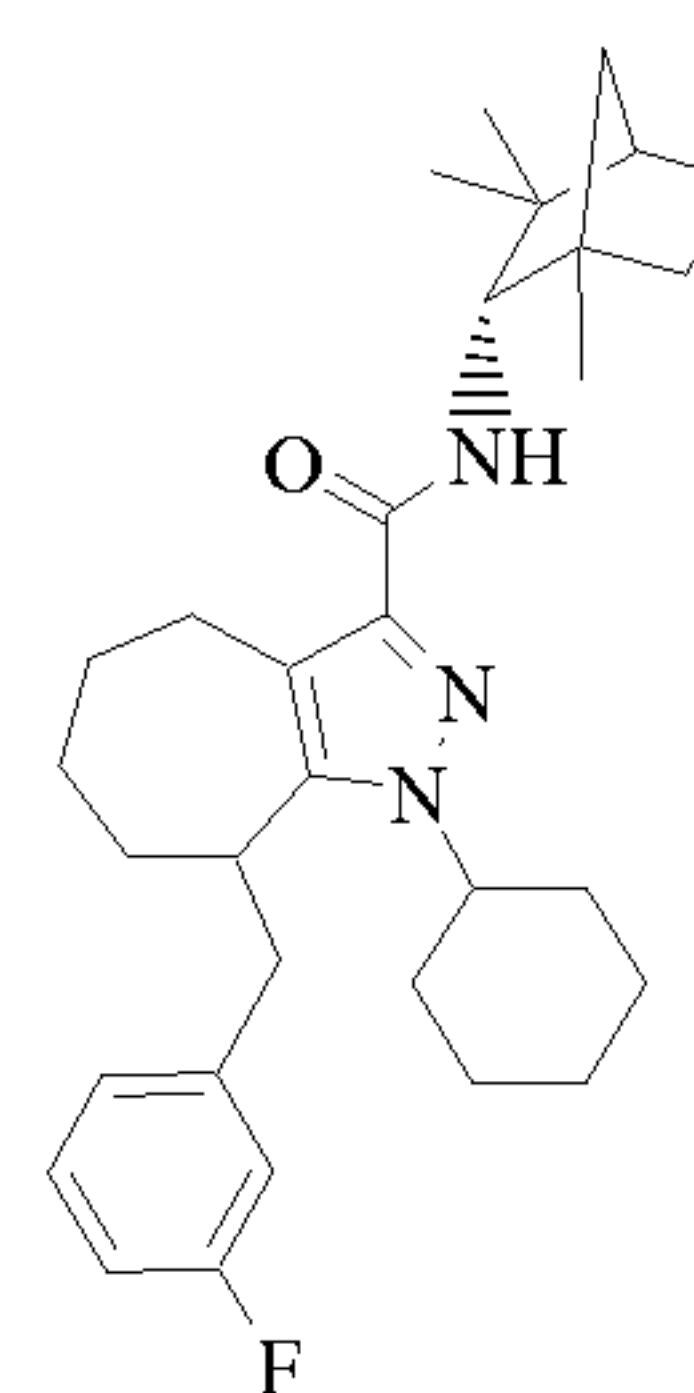
Cpd 44
