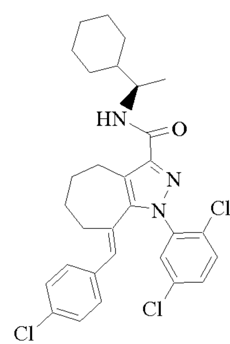
Cpd 196
