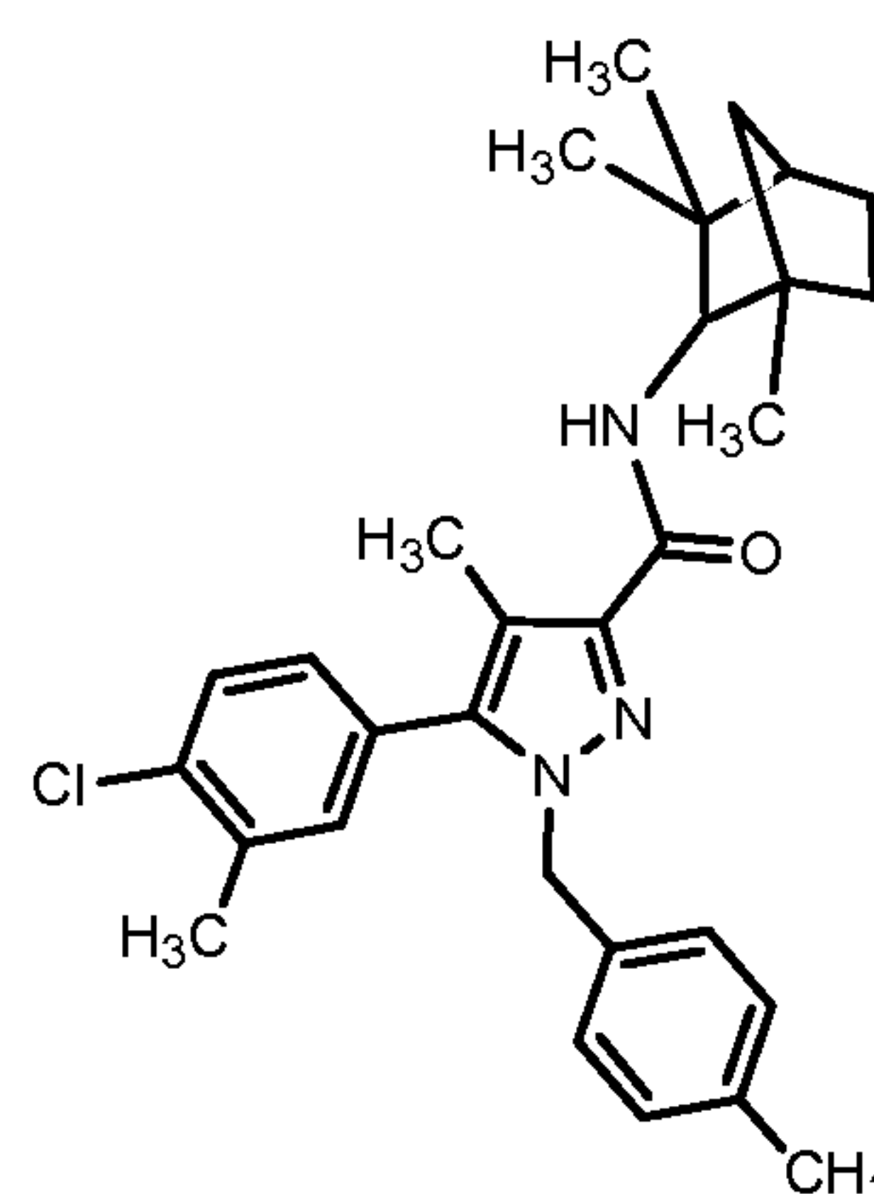
SR 144528
