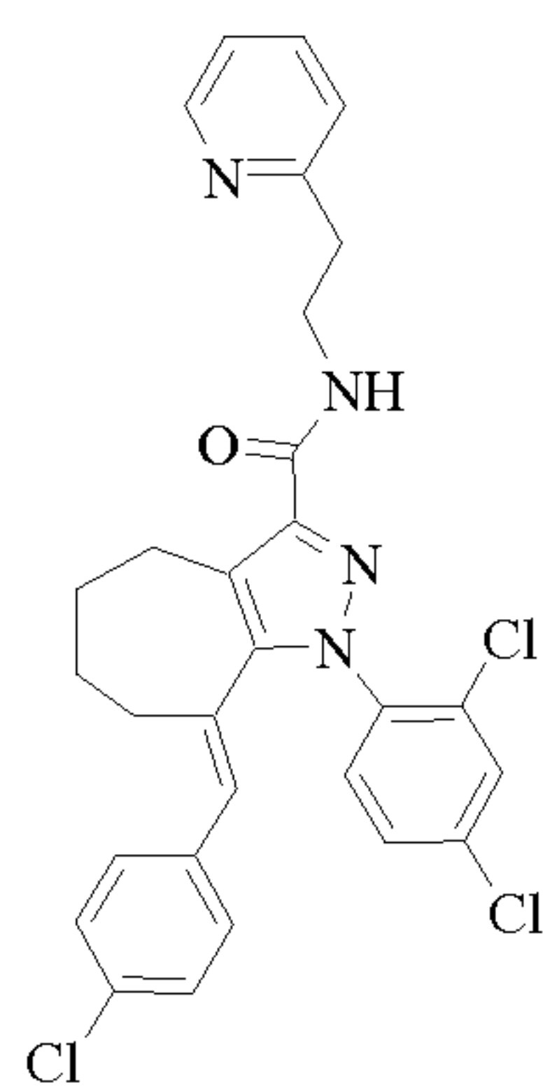
Cpd 157
