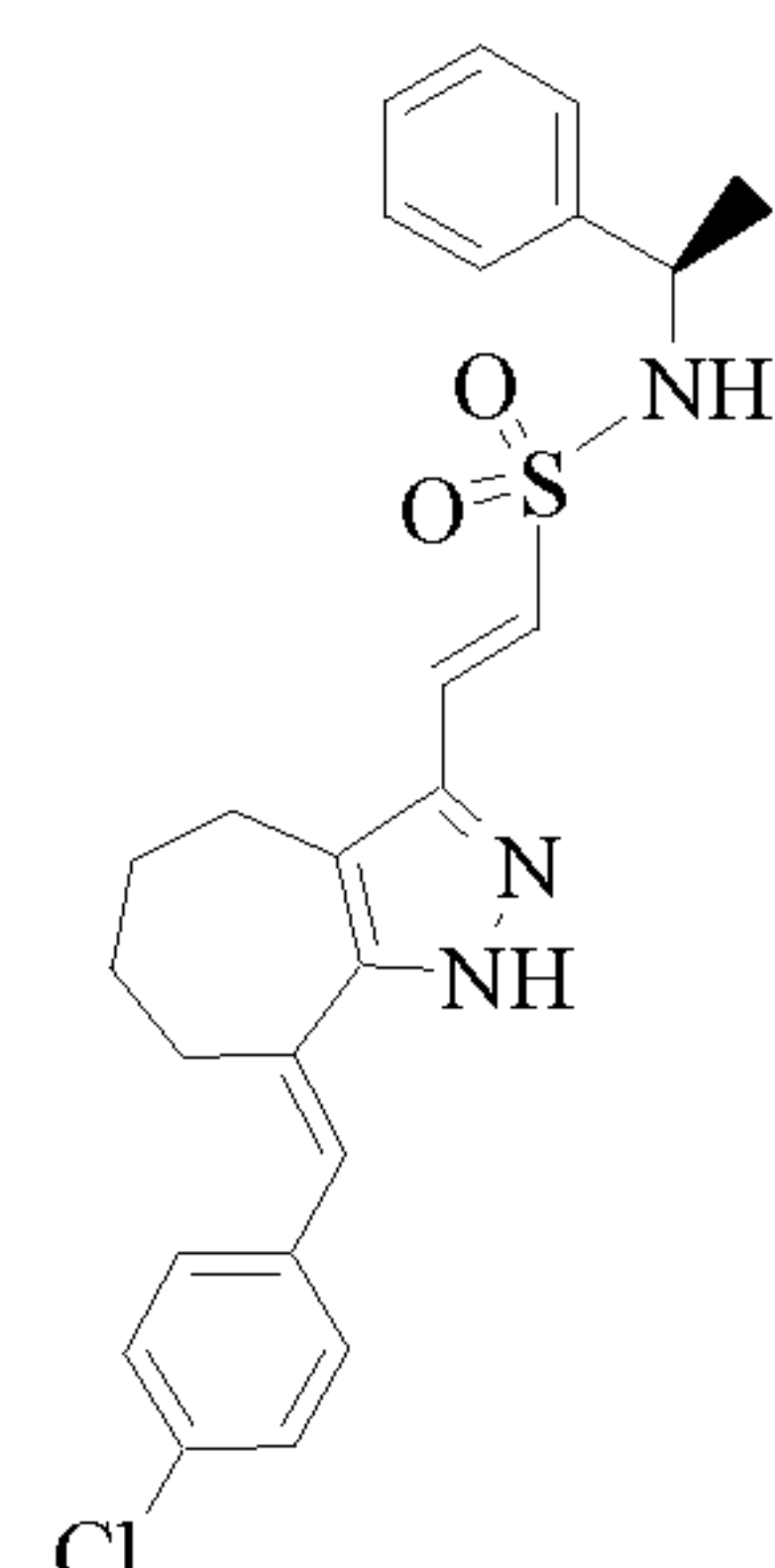
Cpd 236
