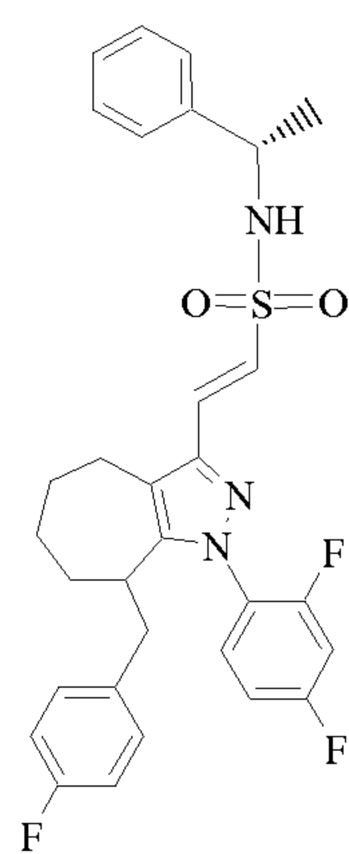
Cpd 107
