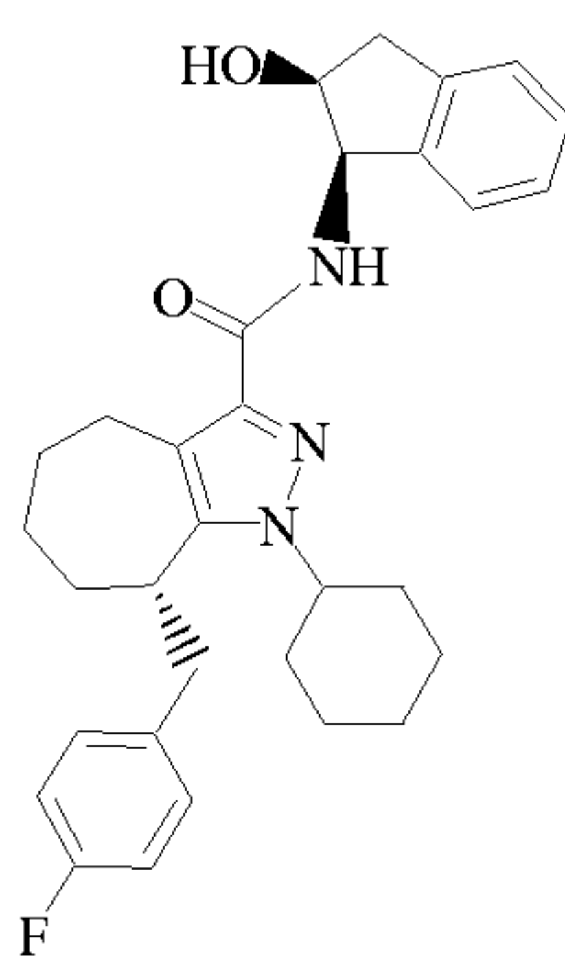
Cpd 117
