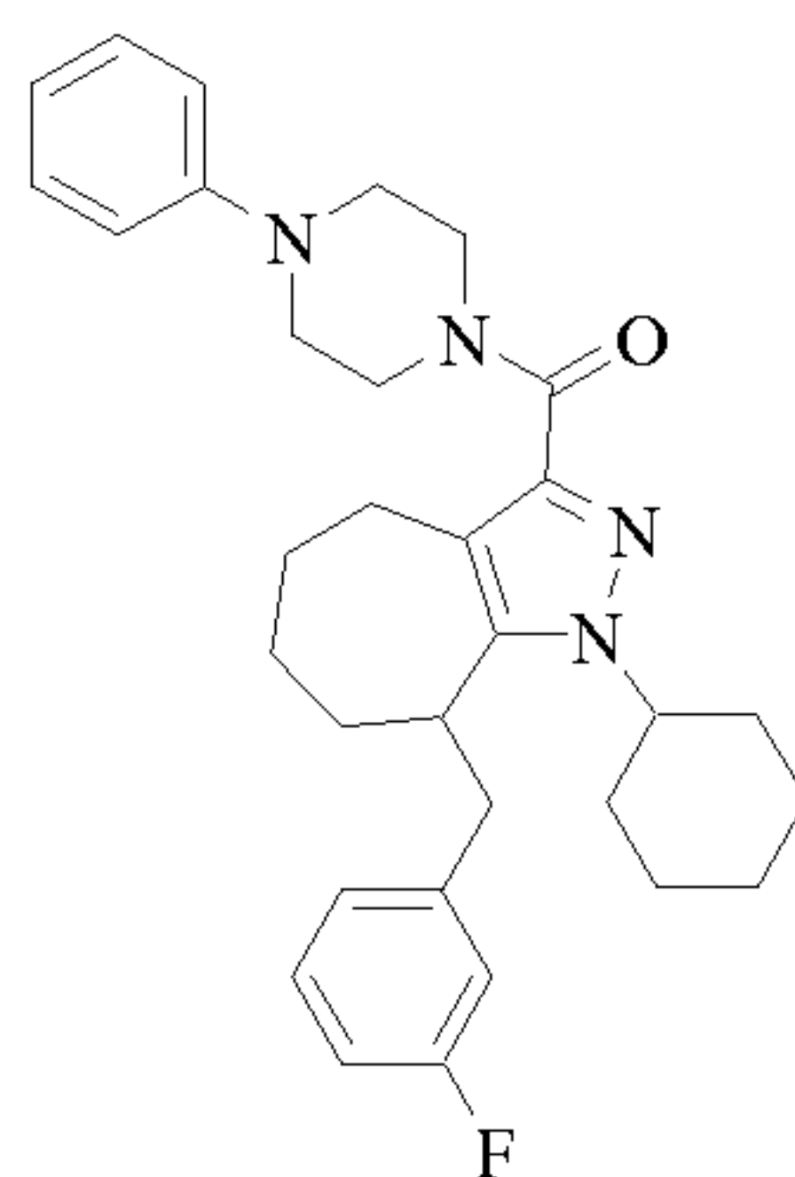
Cpd 54
