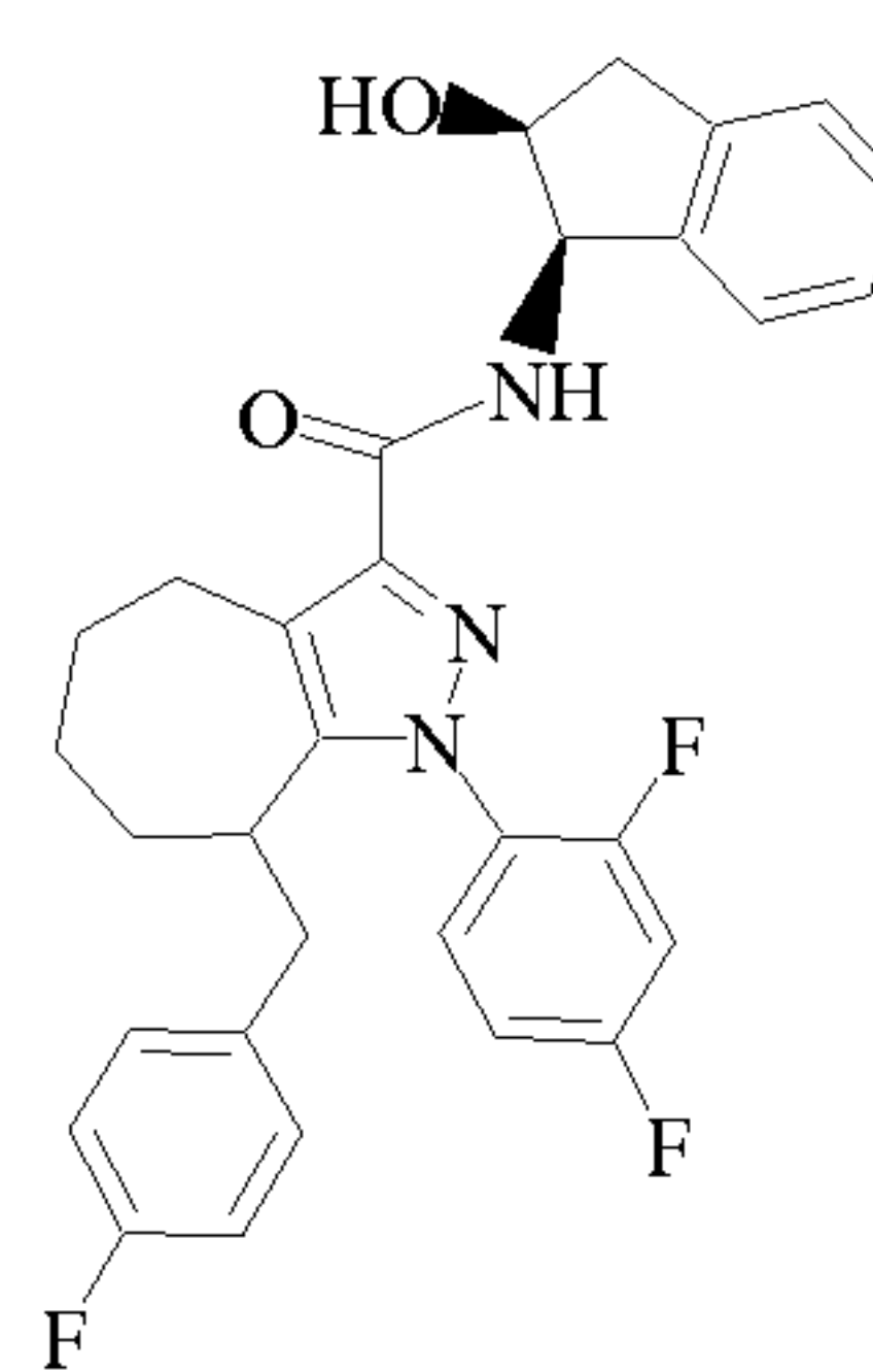
Cpd 115
