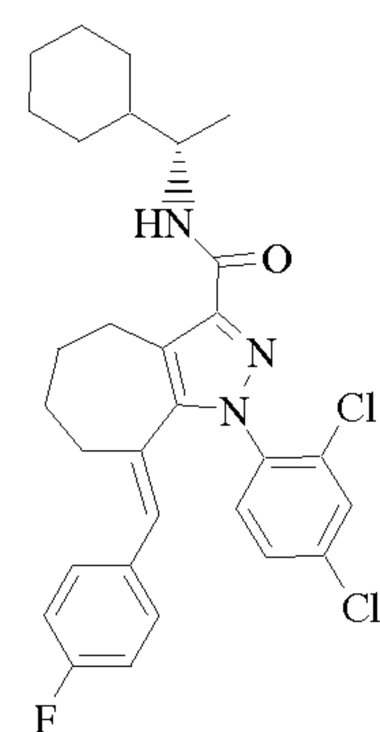
Cpd 148
