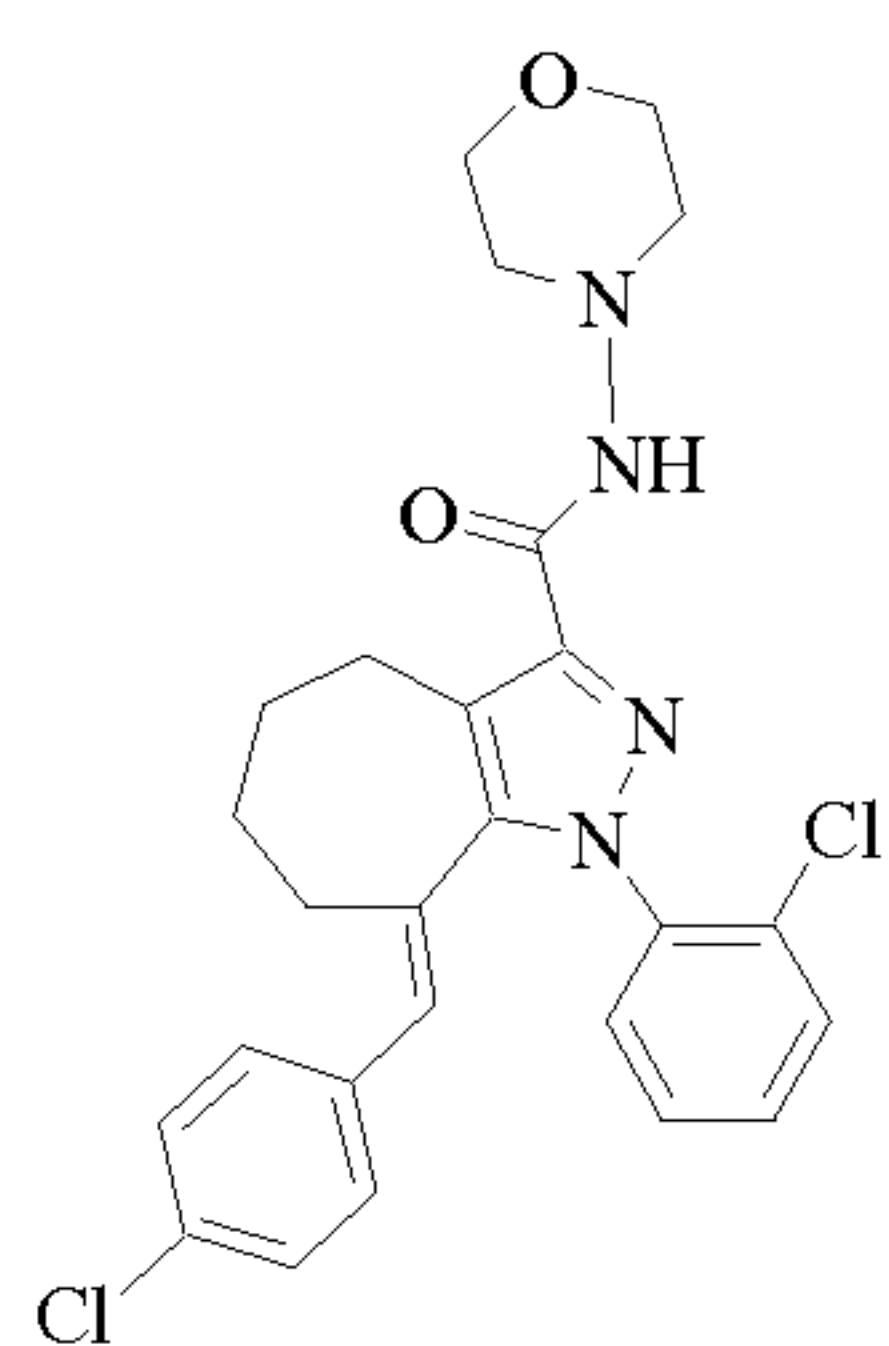
Cpd 194
