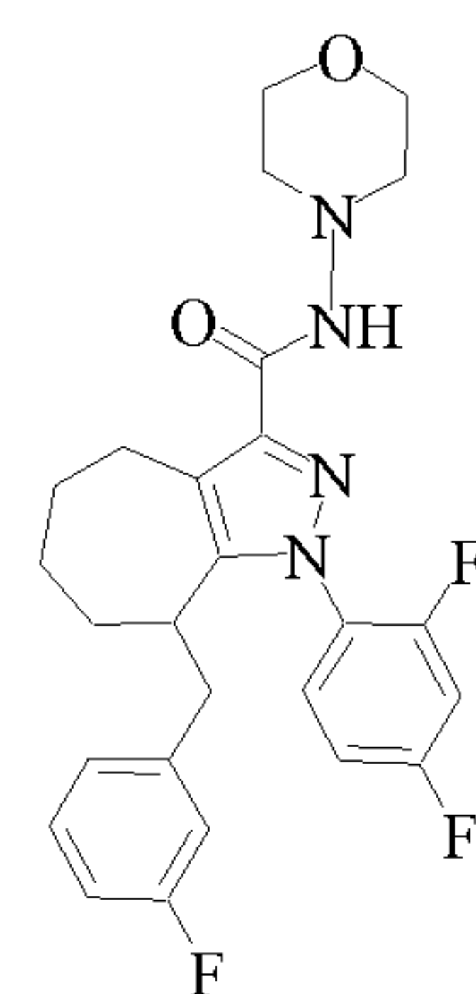
Cpd 116
