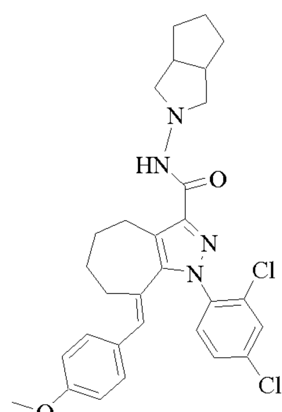
Cpd 226
