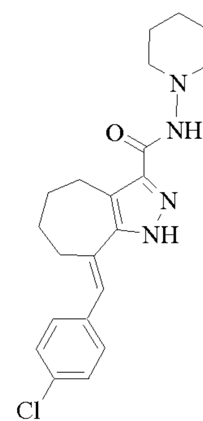
Cpd 144
