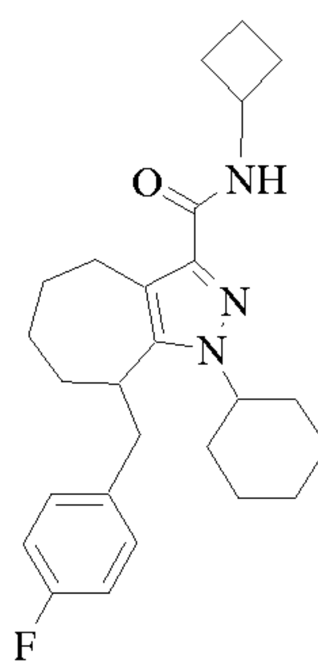
Cpd 57
