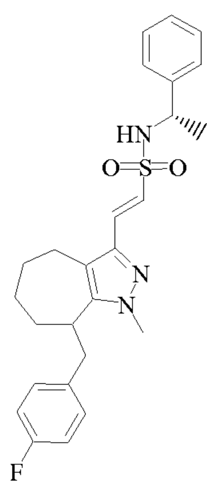
Cpd 101
