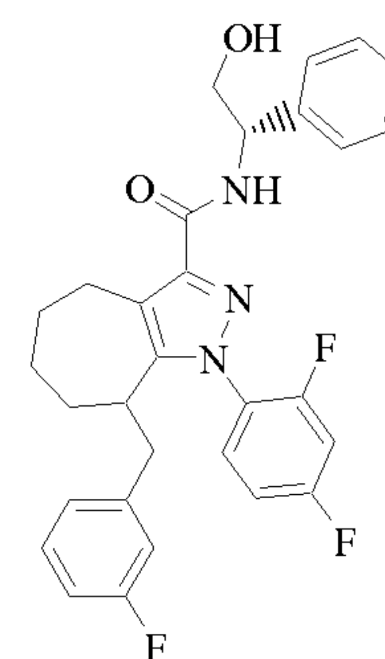
Cpd 168
