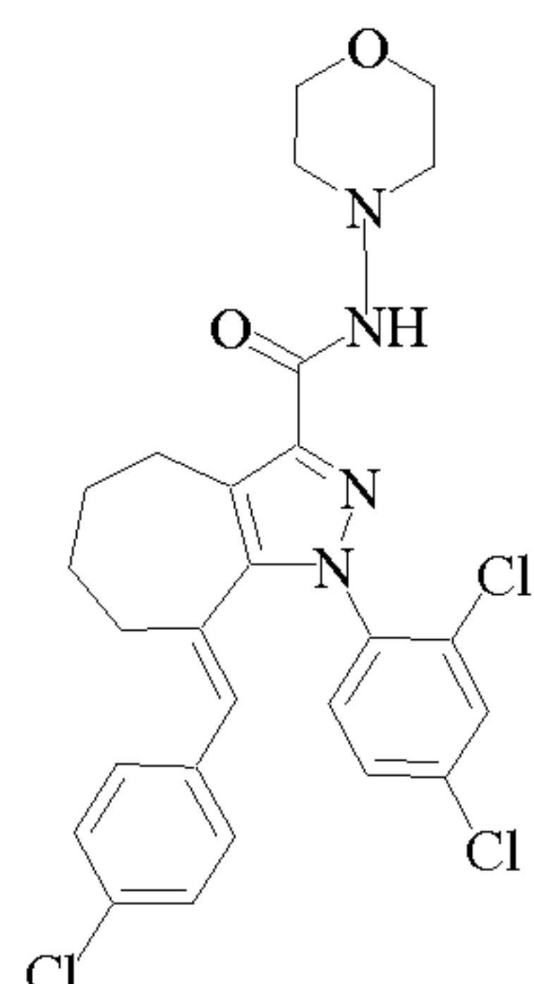
Cpd 134
