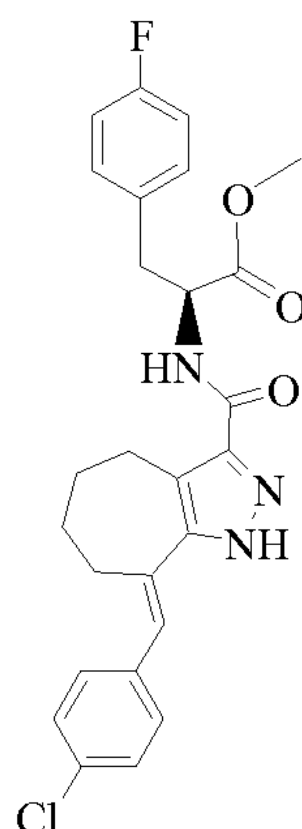
Cpd 238
