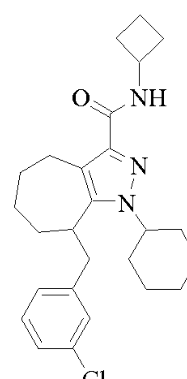
Cpd 36
