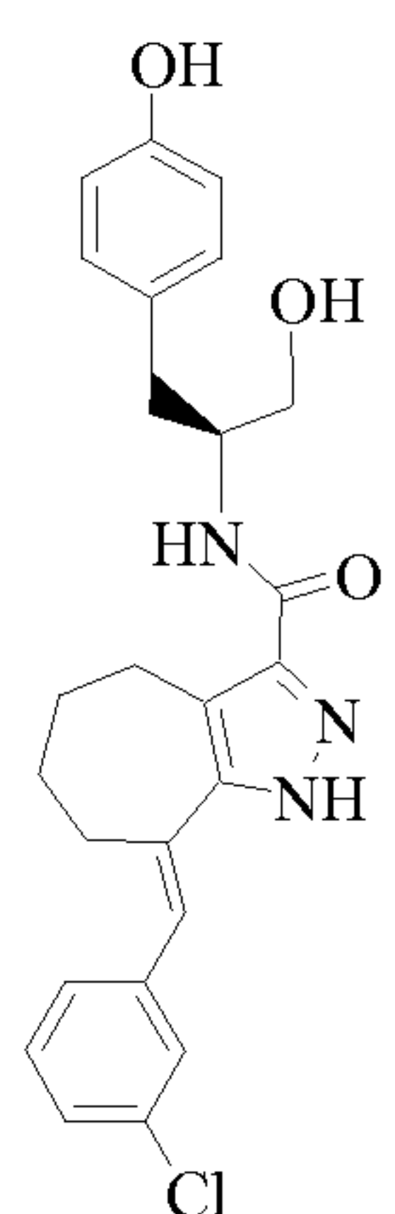
Cpd 246
