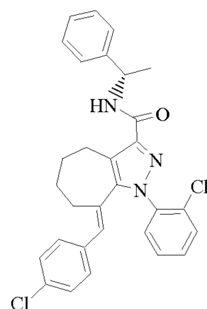
Cpd 191
