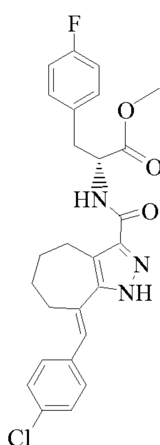
Cpd 247
