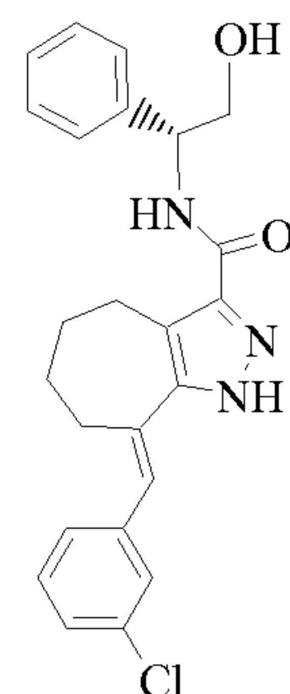
Cpd 235
