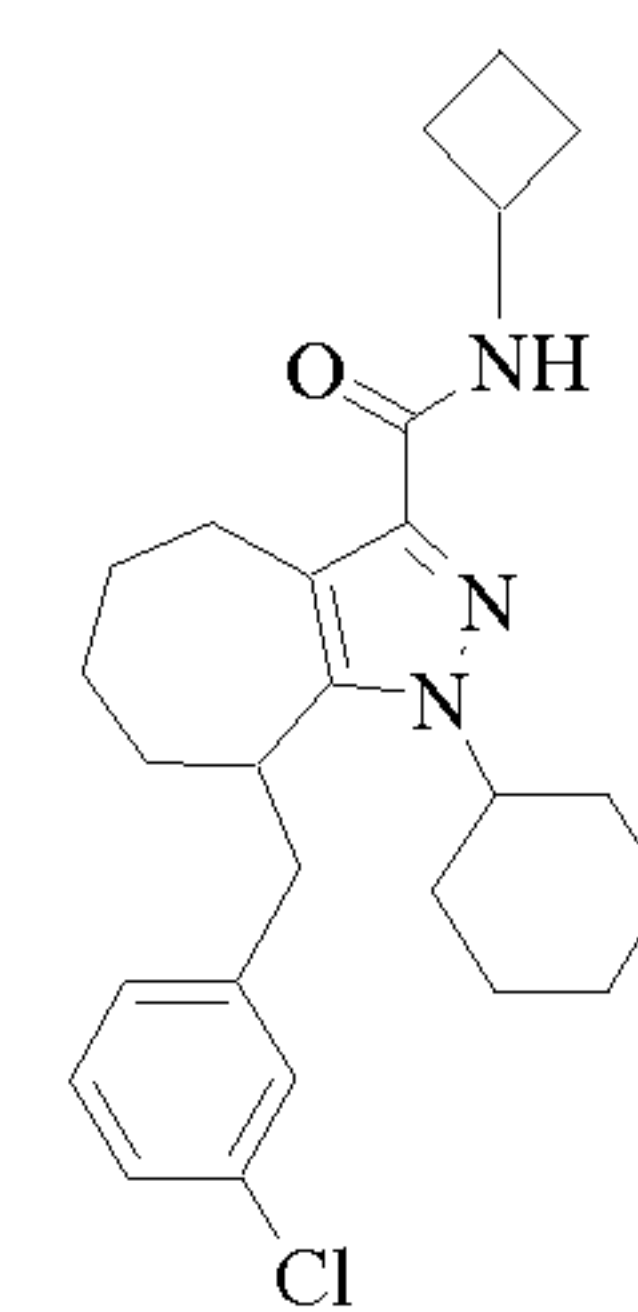
Cpd 24
