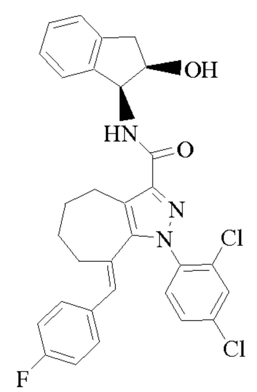
Cpd 204
