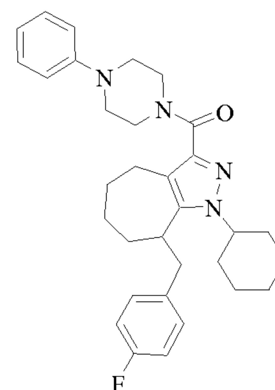
Cpd 60
