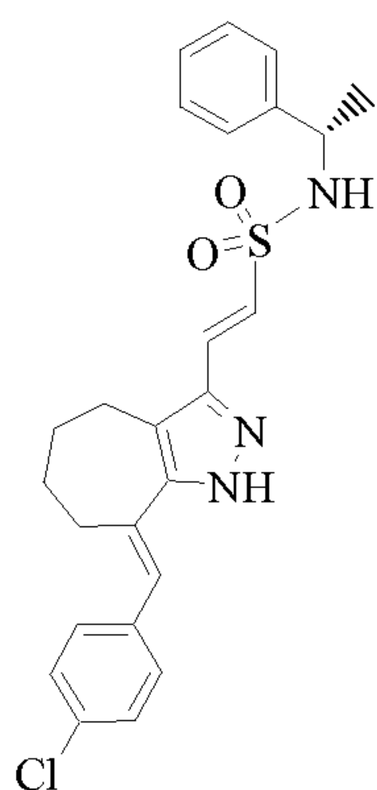
Cpd 233
