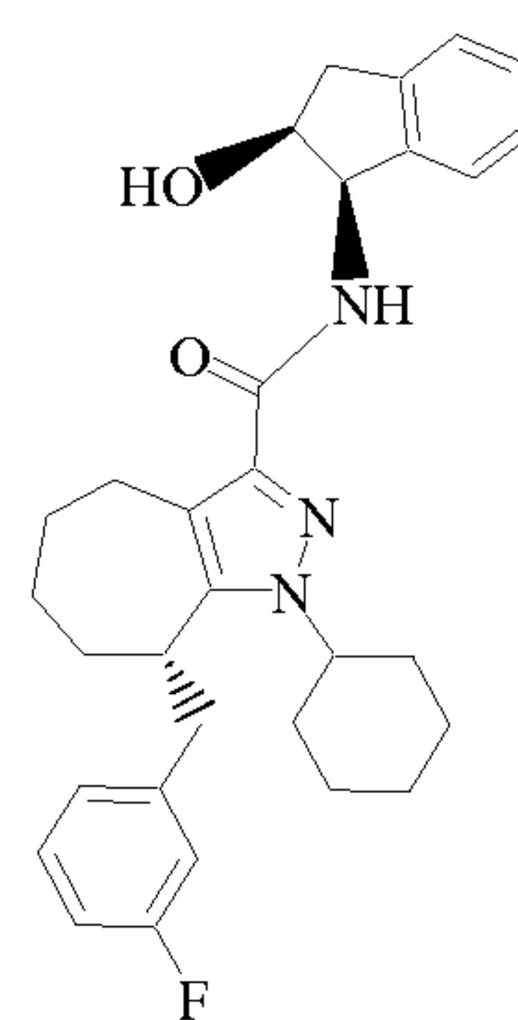
Cpd 115
