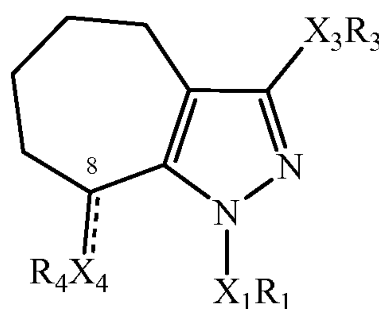
(Ia)
