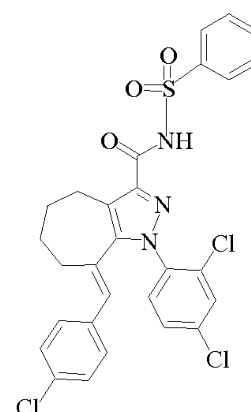
Cpd 136
