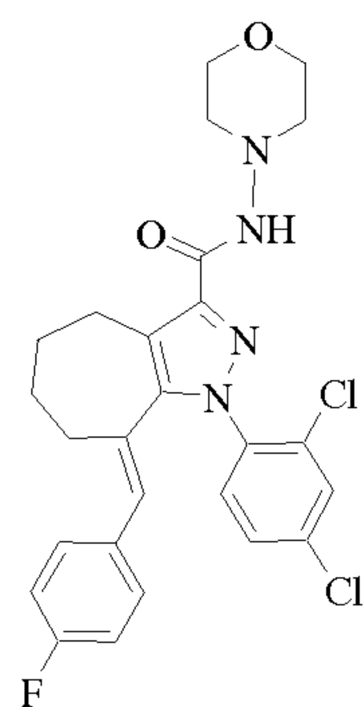
Cpd 151
