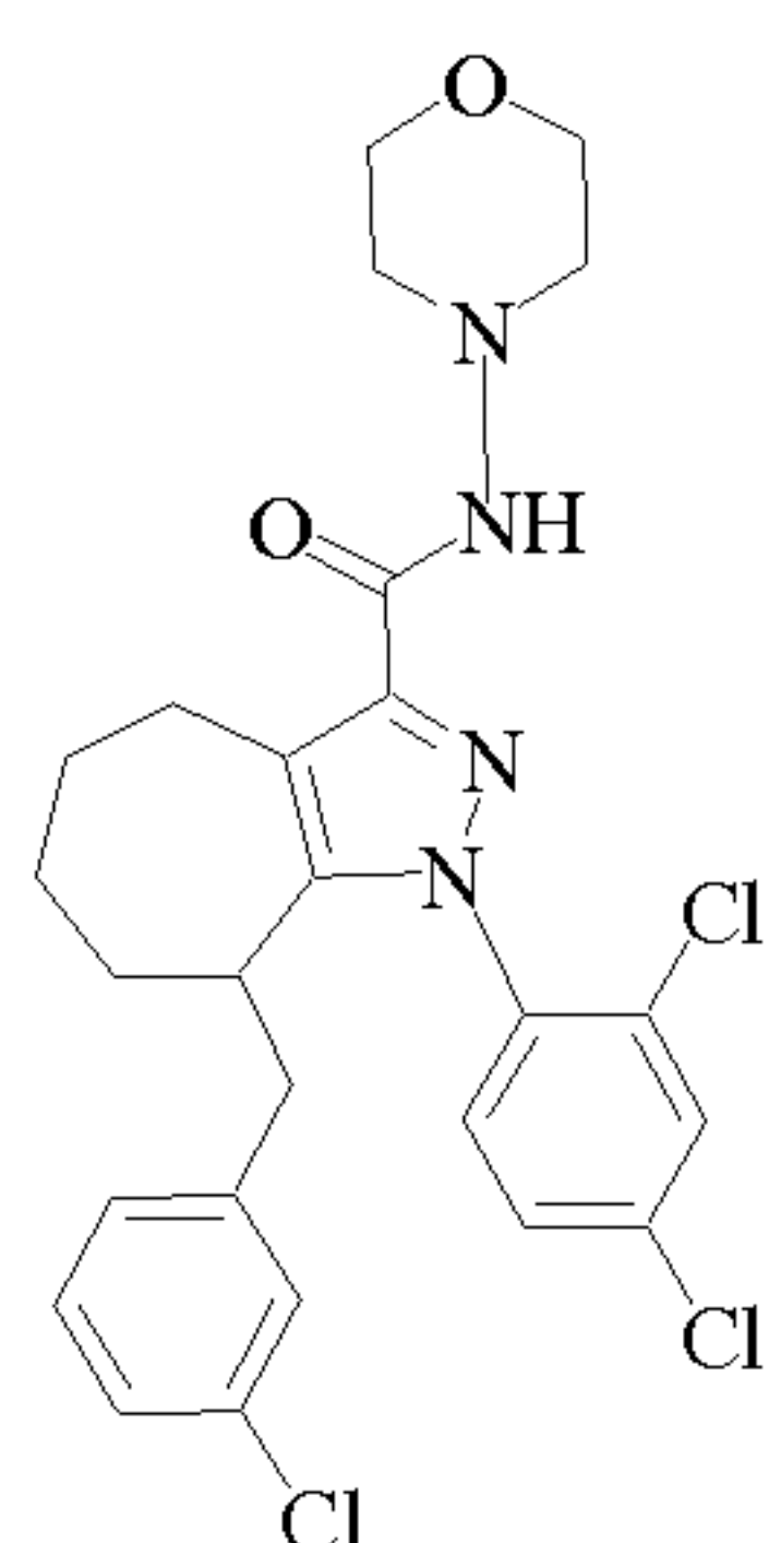
Cpd 117
