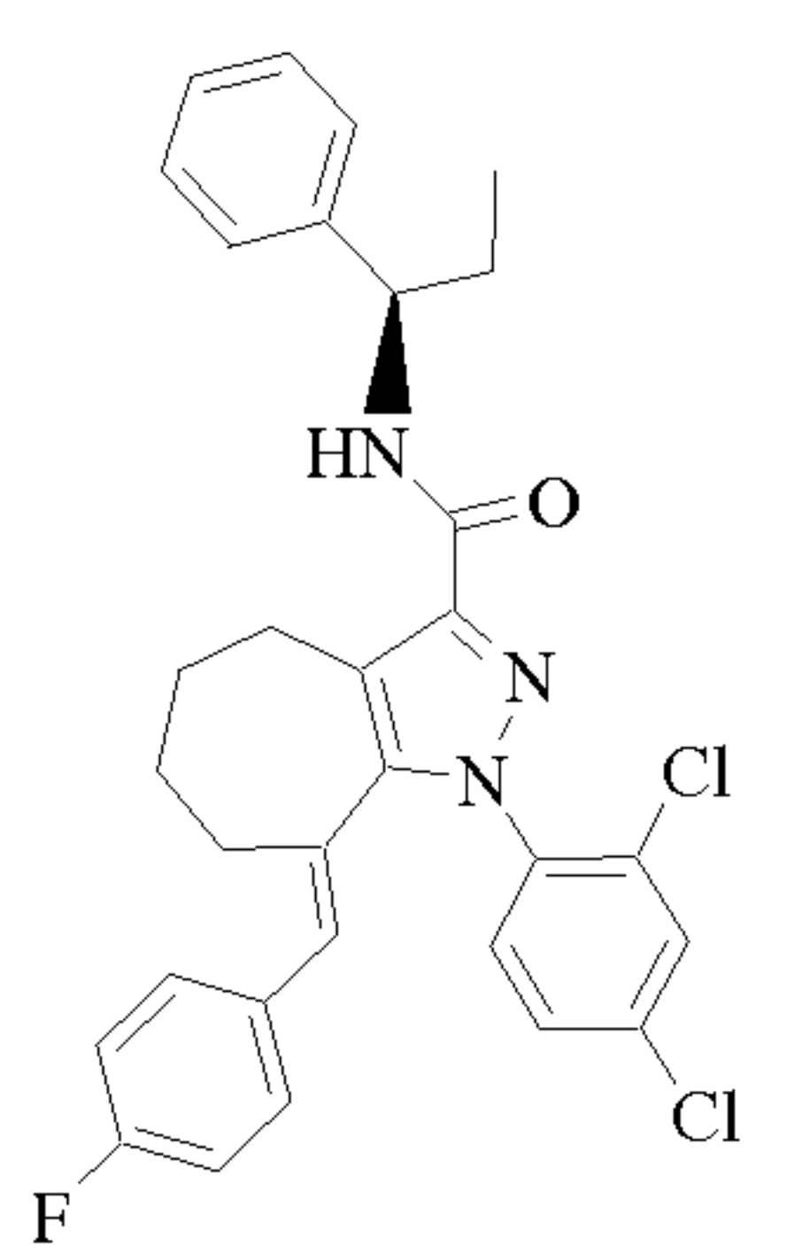
Cpd 202
