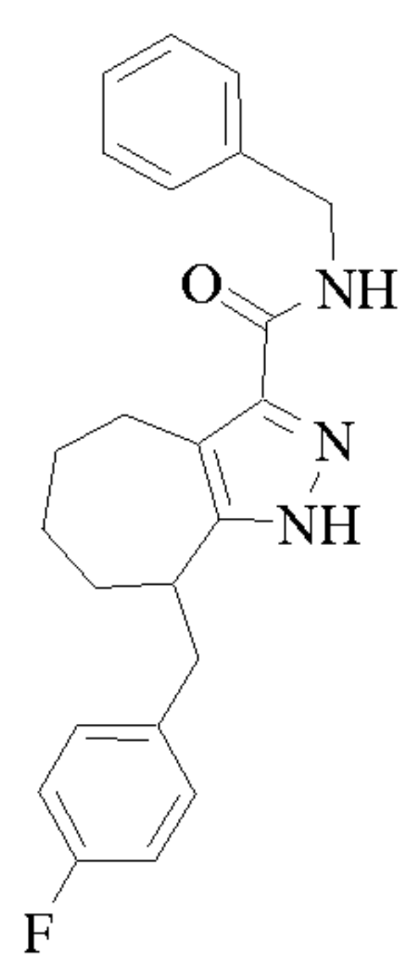
Cpd 129
