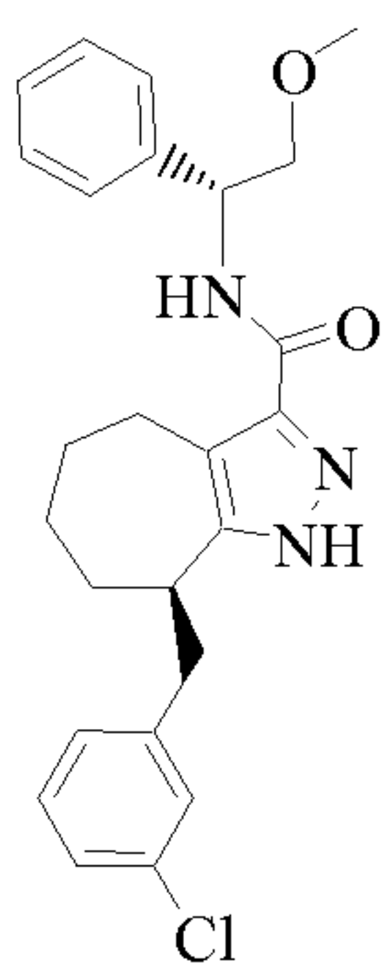
Cpd 254
