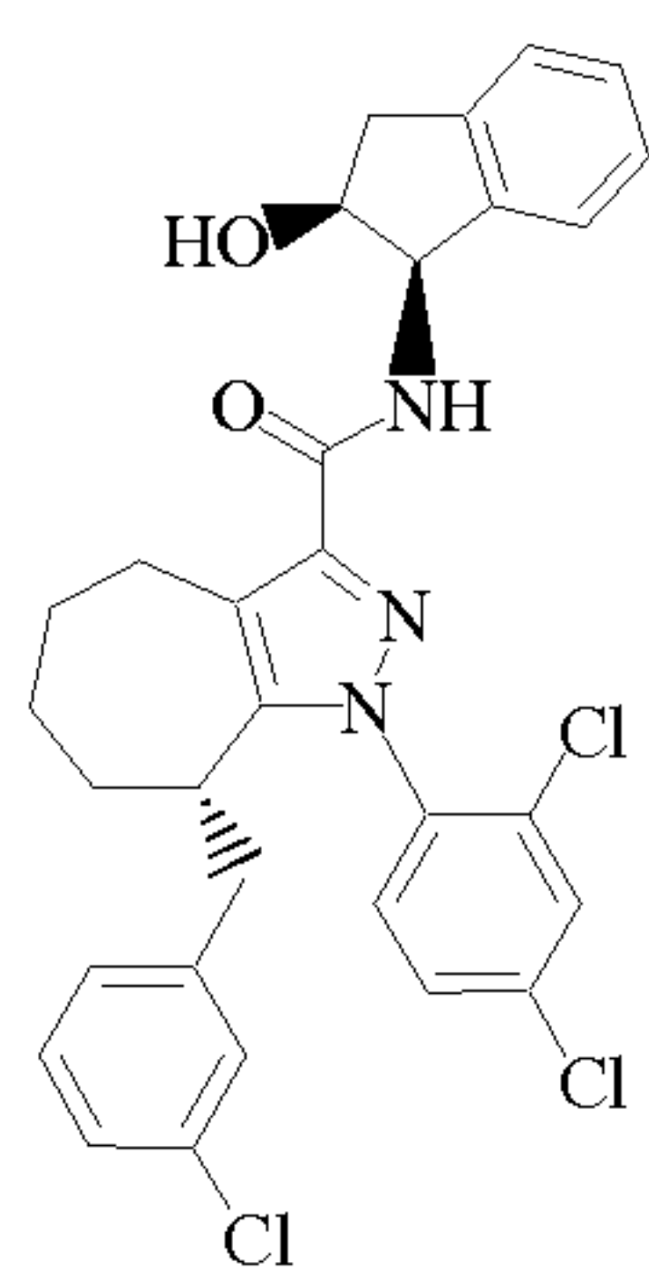
Cpd 113
