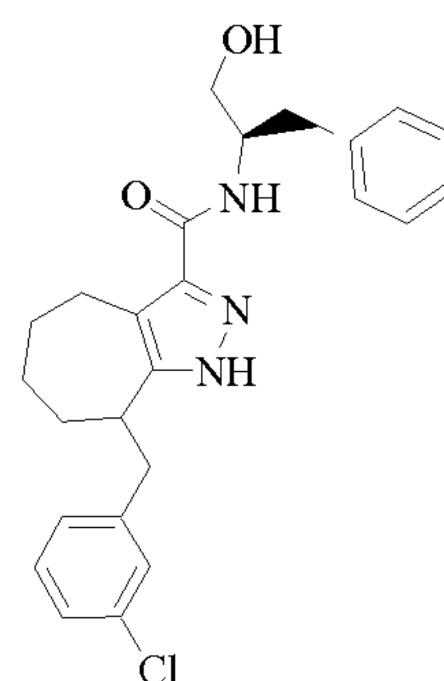
Cpd 167
