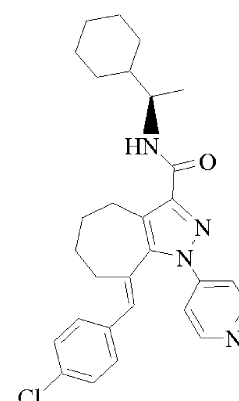
Cpd 180
