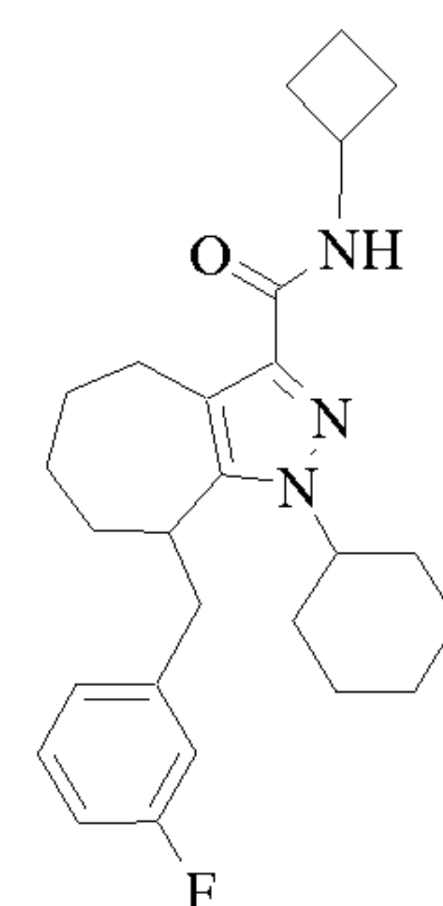
Cpd 39
