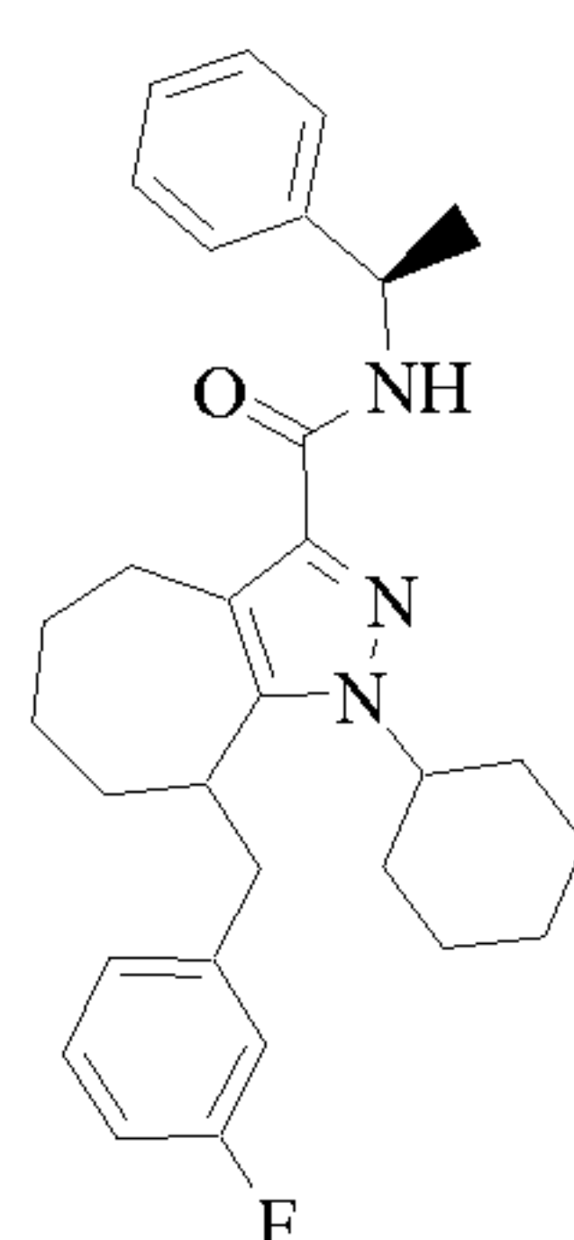
Cpd 174
