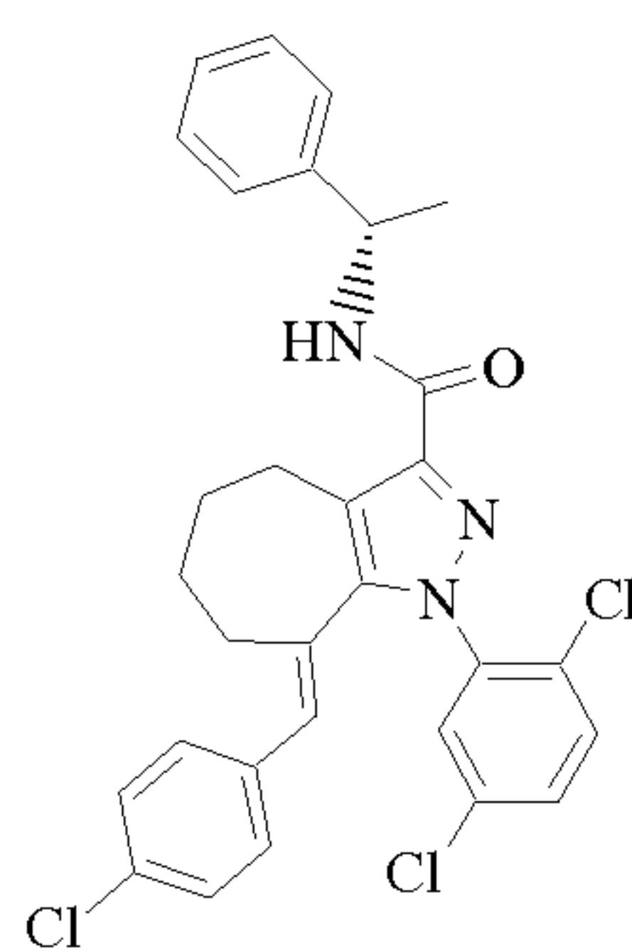
Cpd 198
