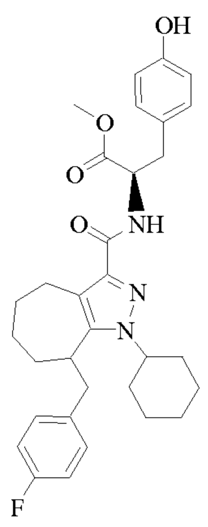
Cpd 83
