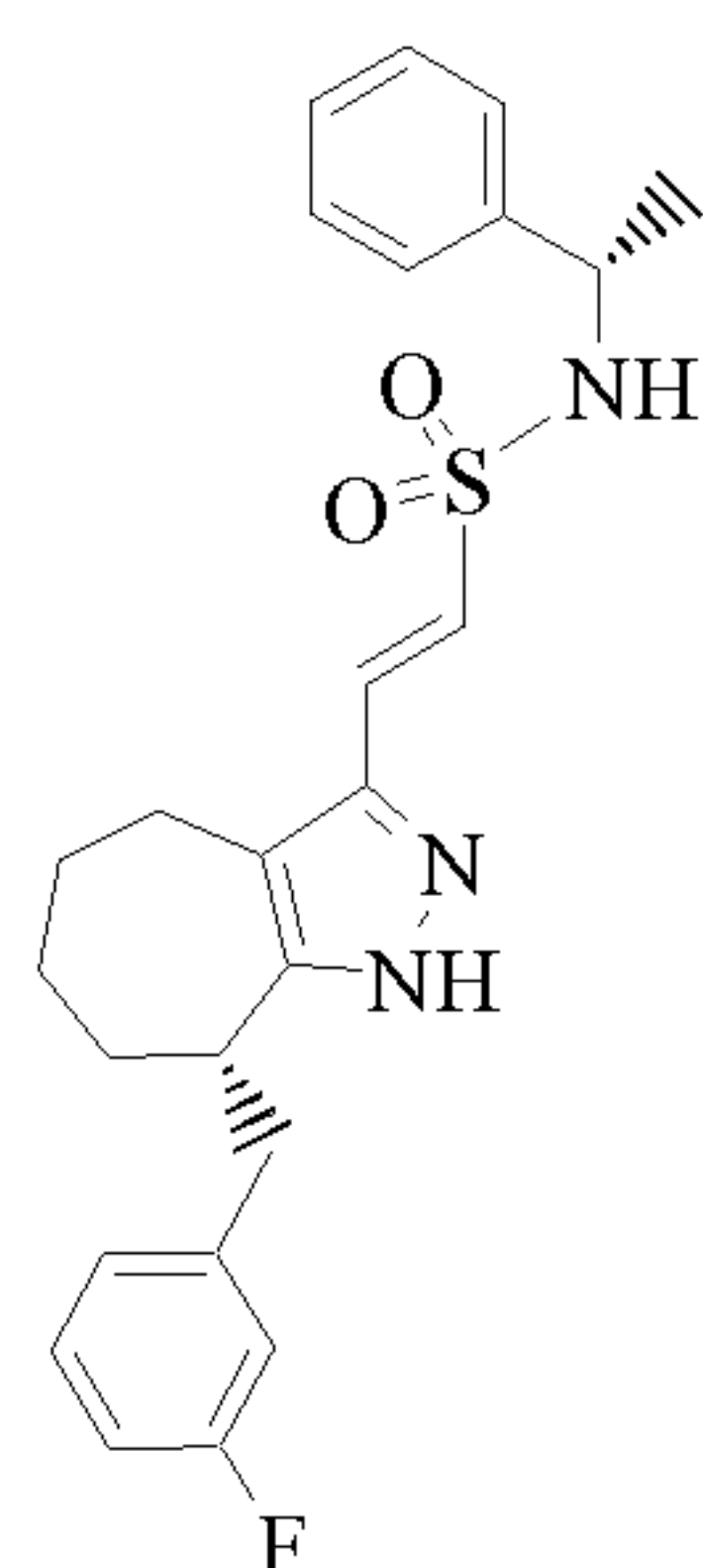
Cpd 233
