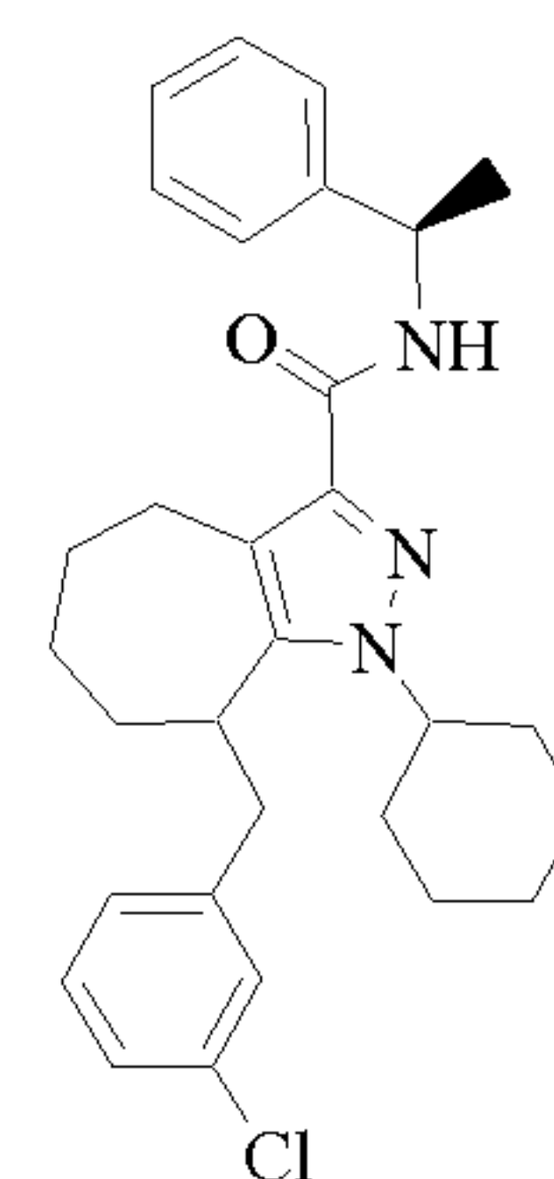
Cpd 4
