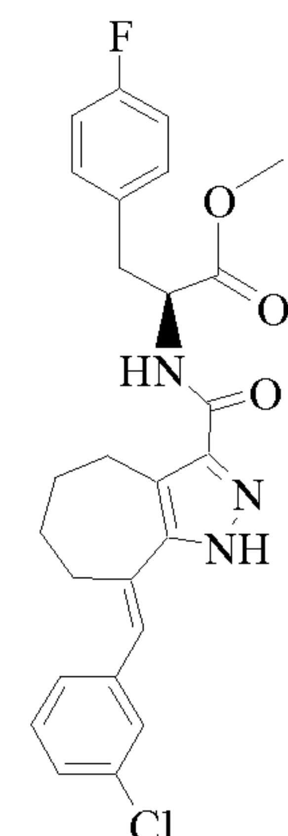
Cpd 240
