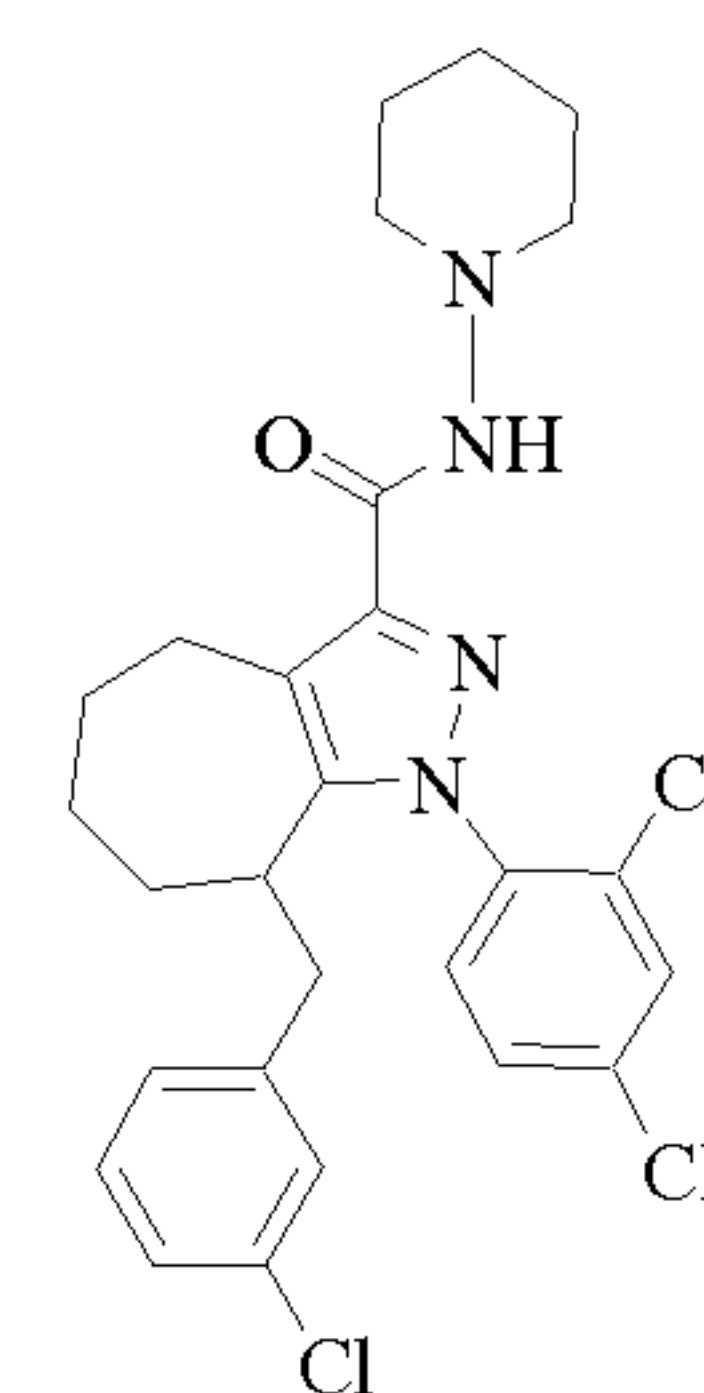
Cpd 24
