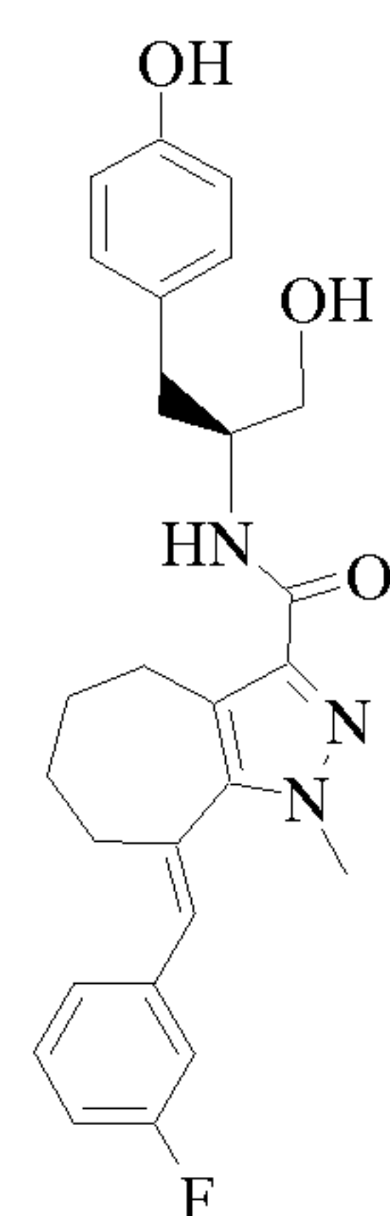
Cpd 244
