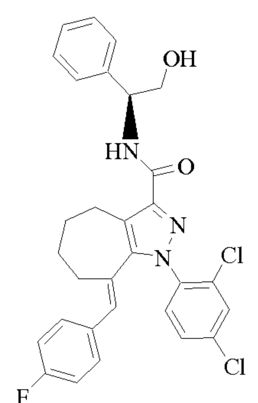
Cpd 204
