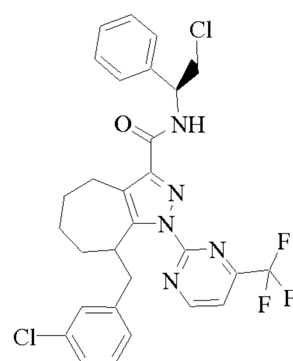
Cpd 179
