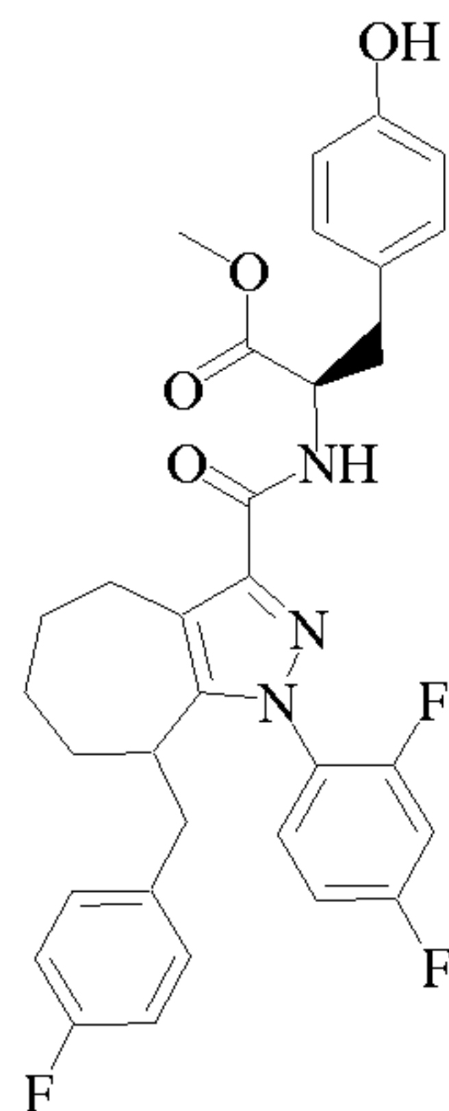
Cpd 98
