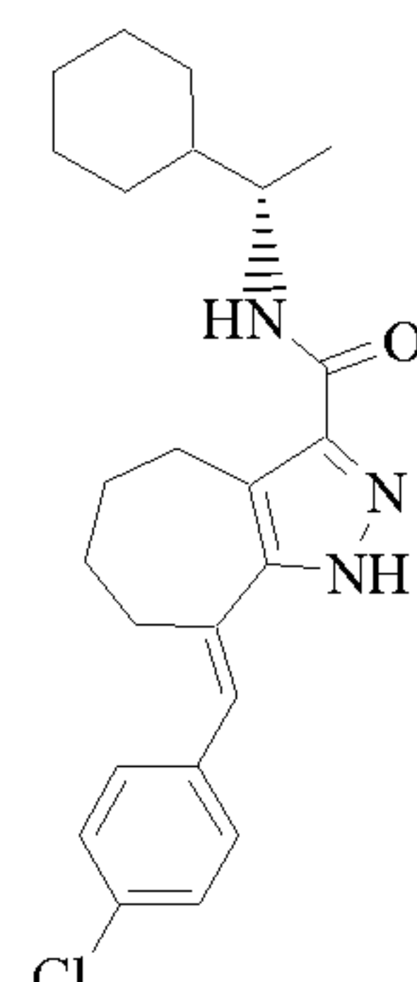
Cpd 143
