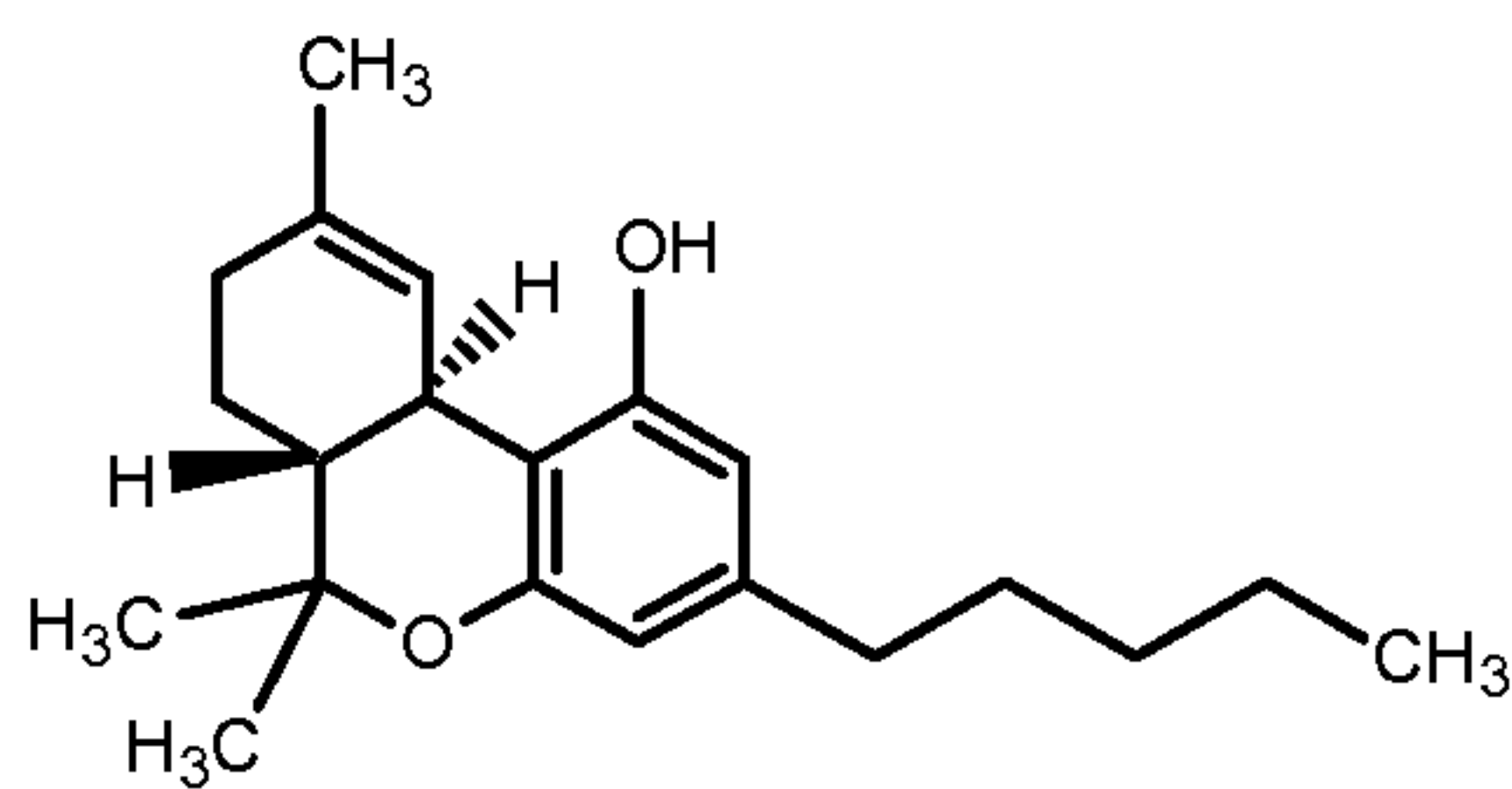
THC
