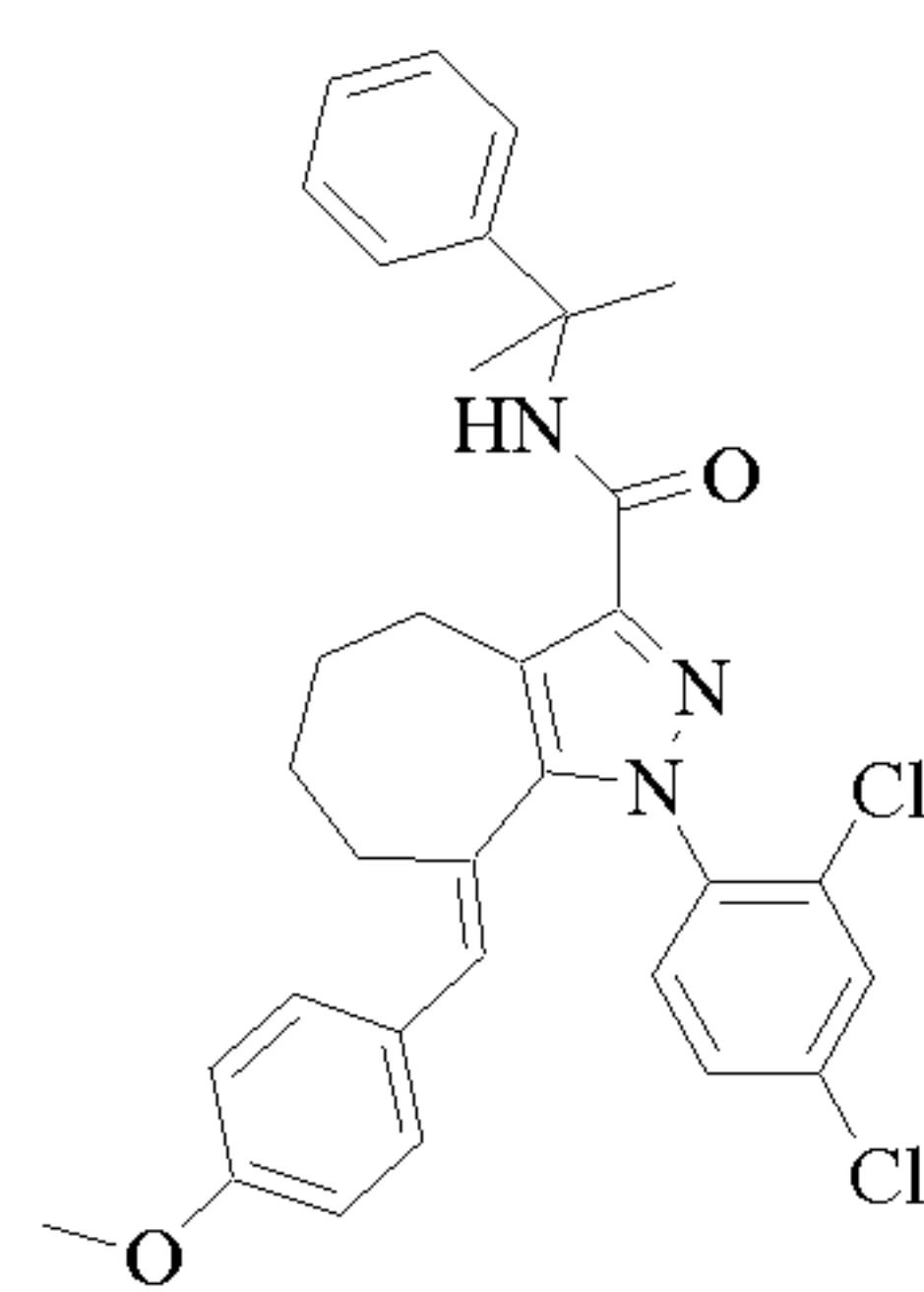
Cpd 211
