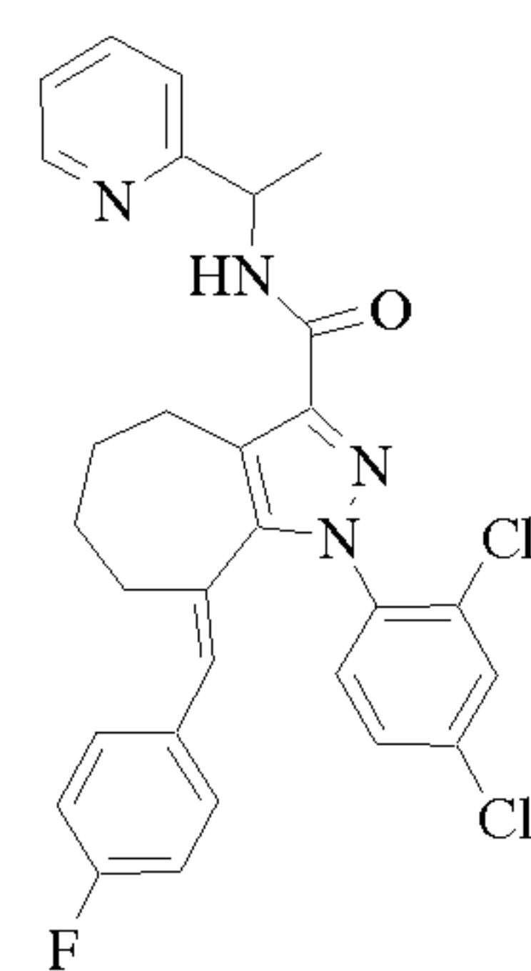
Cpd 224
