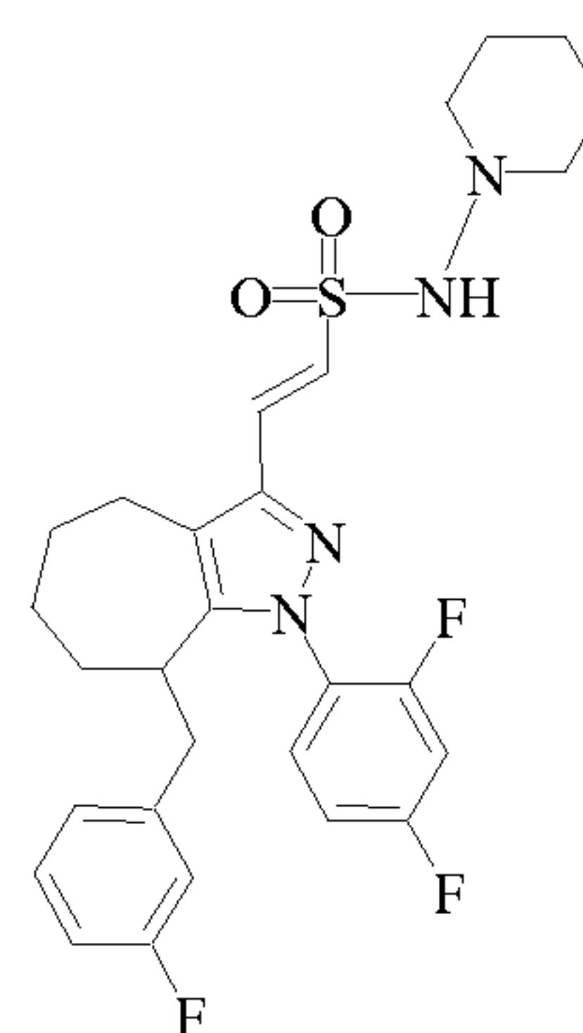
Cpd 119
