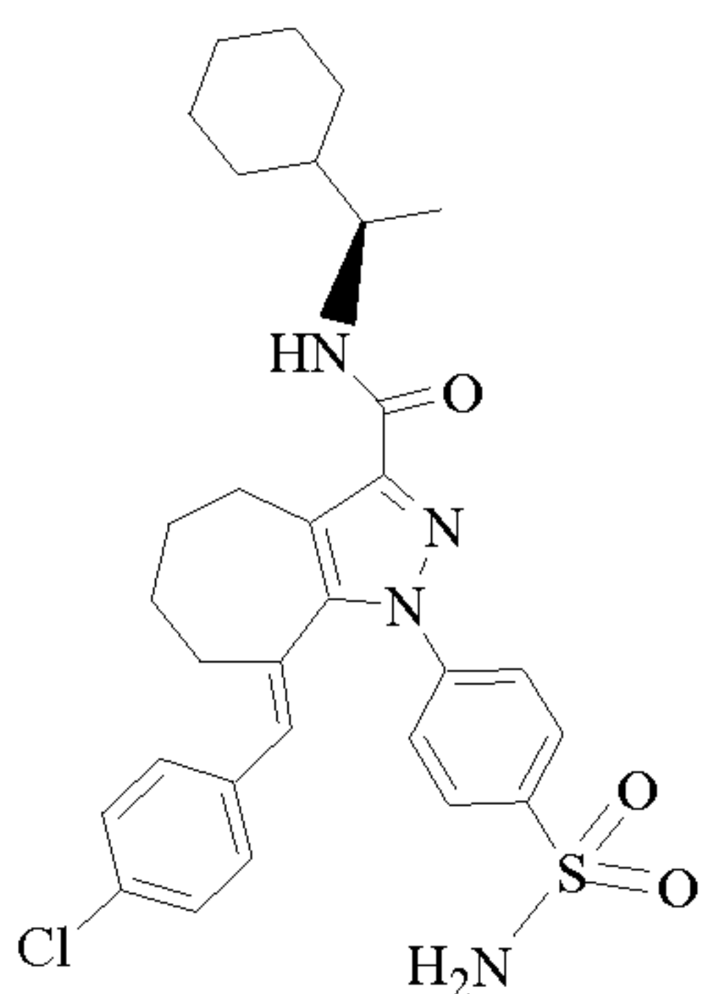
Cpd 185
