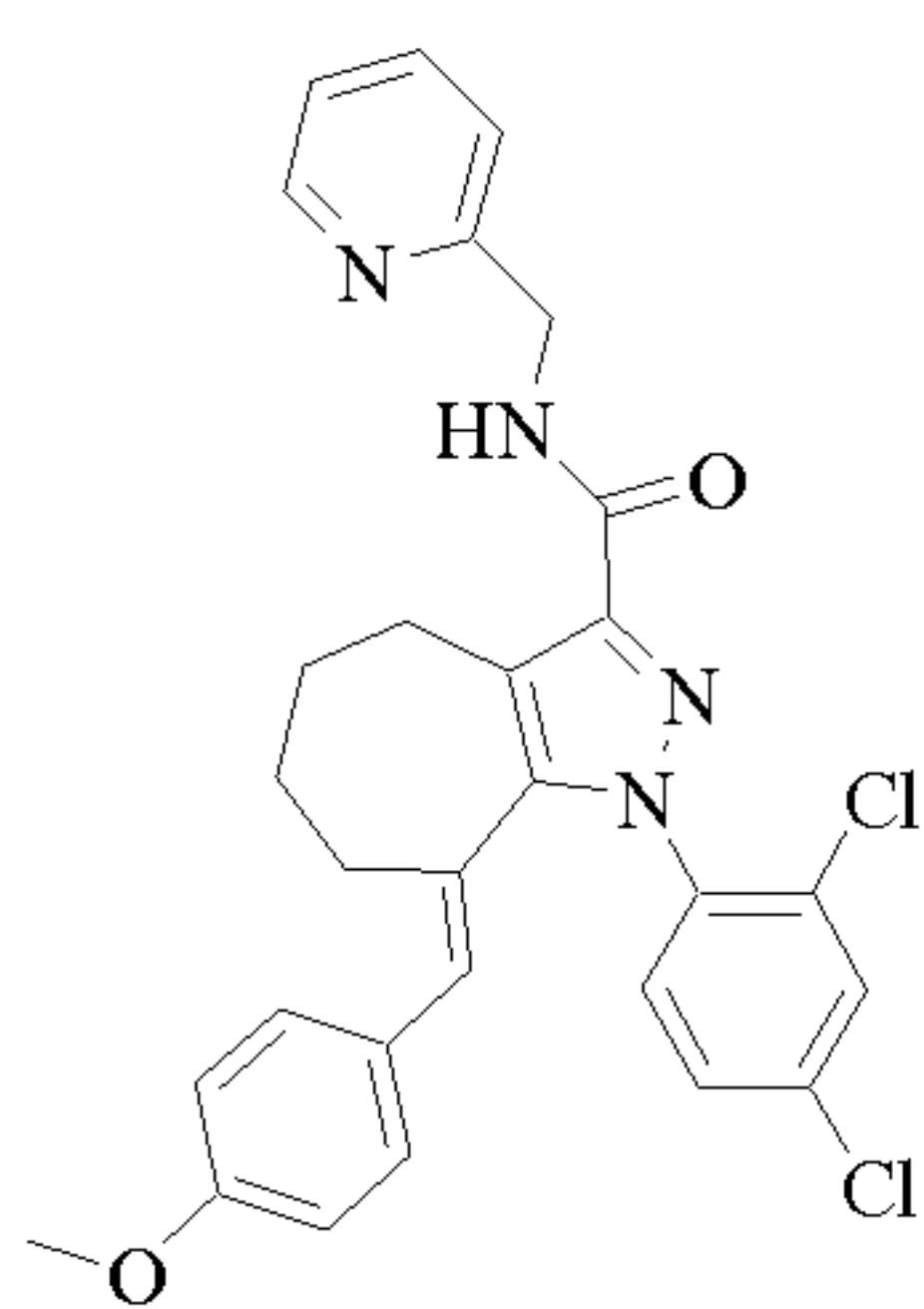
Cpd 210
