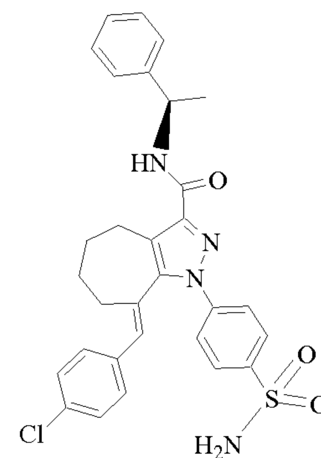
Cpd 184
