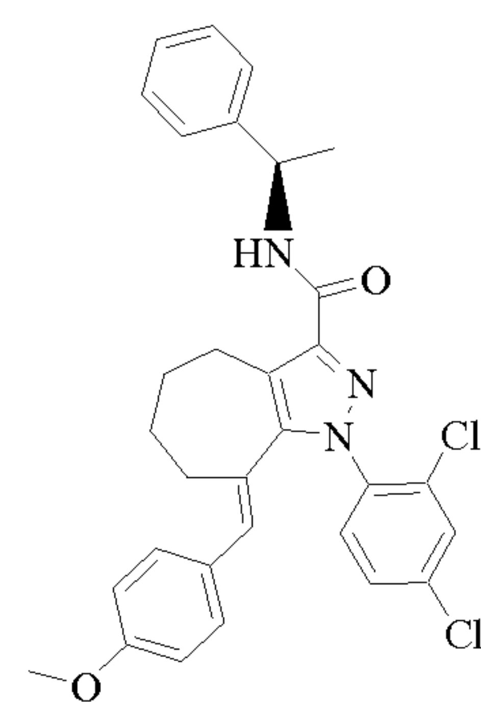
Cpd 212
