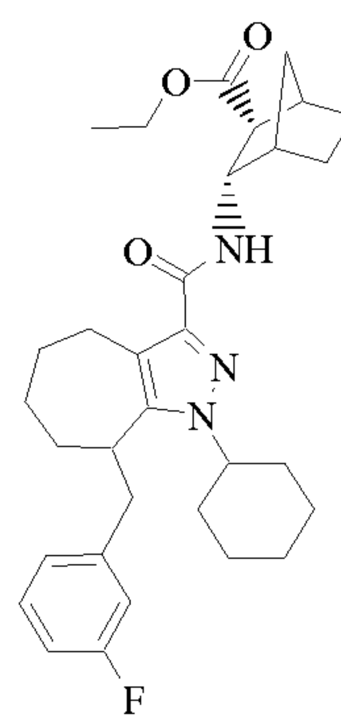
Cpd 101
