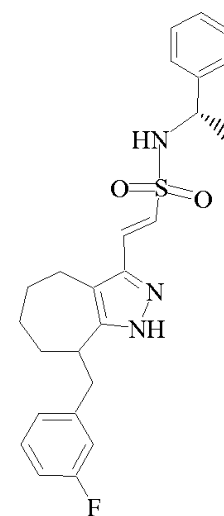
Cpd 96
