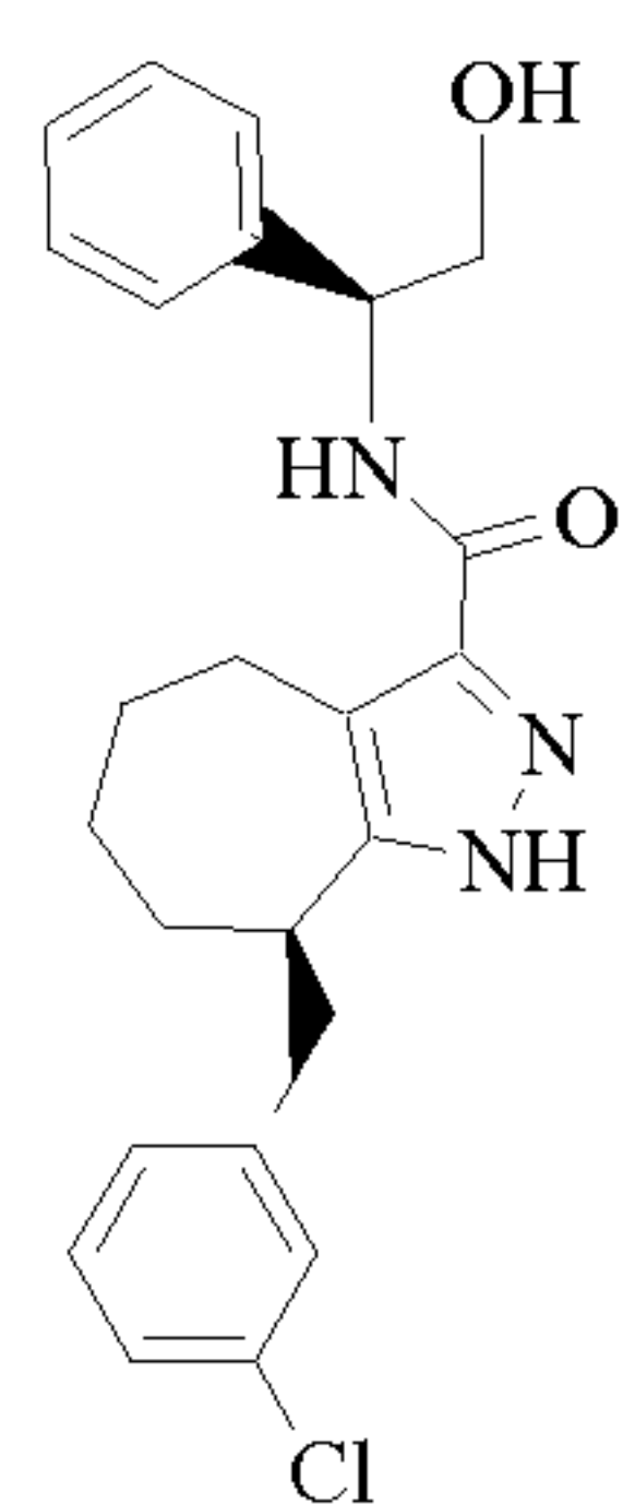
Cpd 226
