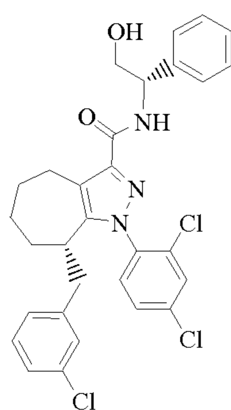
Cpd 162
