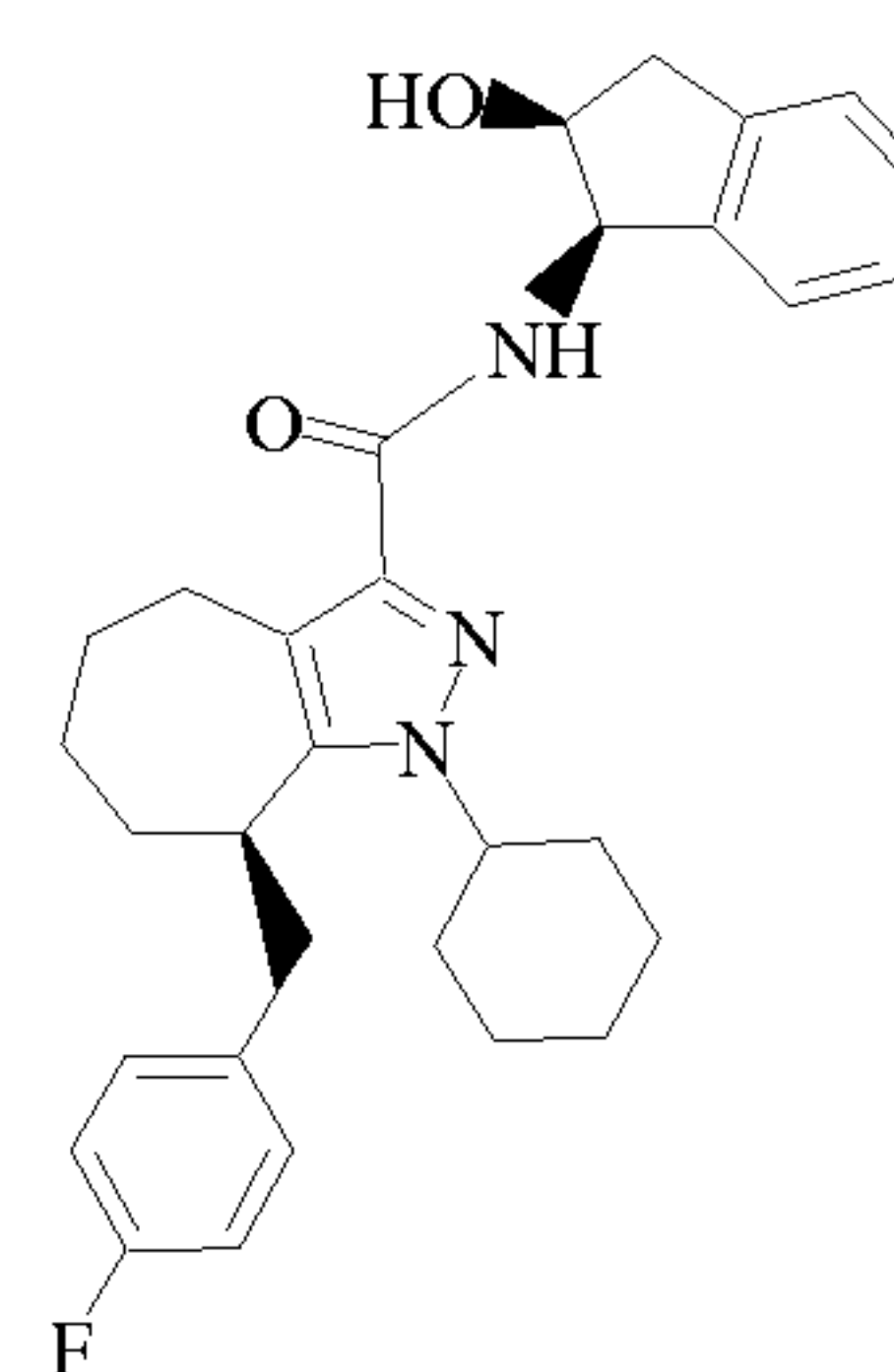
Cpd 120
