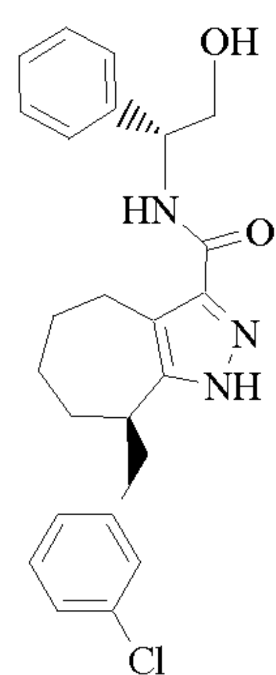
Cpd 225
