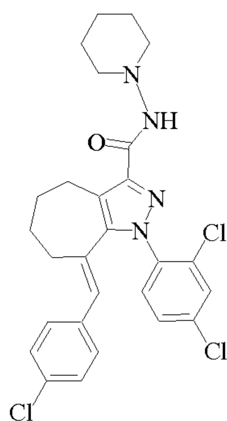
Cpd 133
