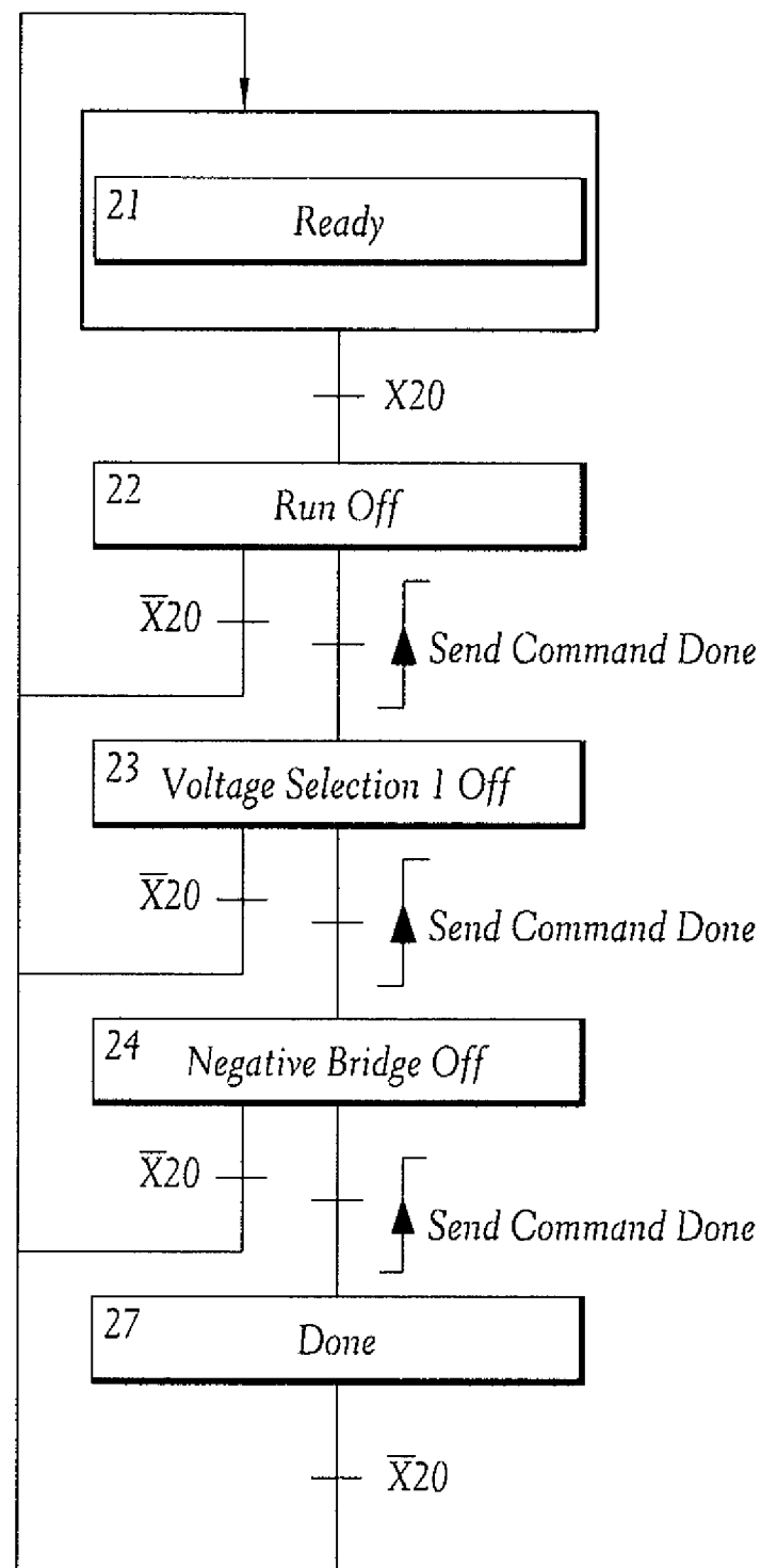
FIG. 7 Ready SFC
