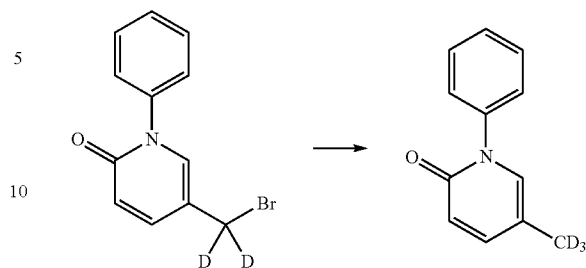
d 3 -5-(Methyl)-1-phenylpyridine-2(1H)-one
