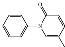
Pirfenidone
