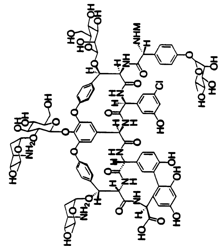
\beta -Avoparcin
