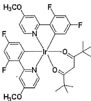
(F_2ppy)_2Ir(tmd)
