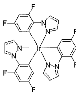
Ir(dfppz)_3
