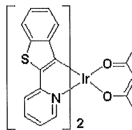
Btp 2 Ir(acac)
