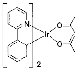
Ir(ppy) 2 (acac)
