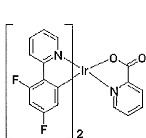
F_2Irpic
