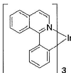
Ir(piq) 3
