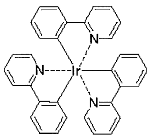
Ir(ppy) 3
