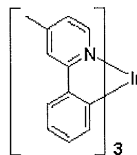
Ir(mpyp) 3
