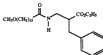
Ethyl \alpha -[[[(12-Methoxy-1-oxododecyl)amino]-methyl]benzenepropanoate
