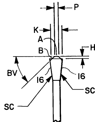
FIG. 3E PRIOR ART
