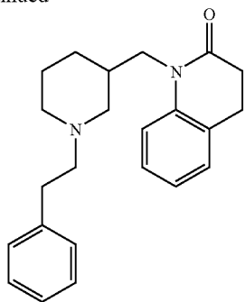
130
