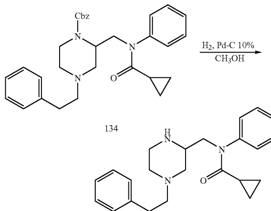
135
