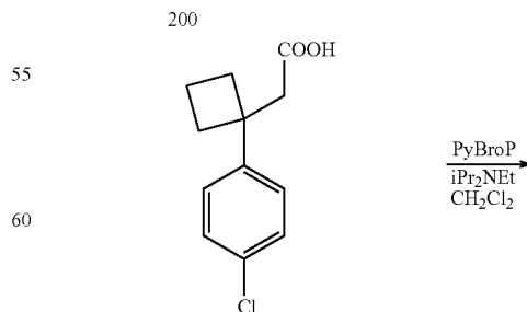
201
