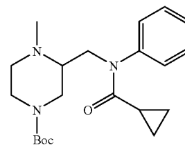
136
