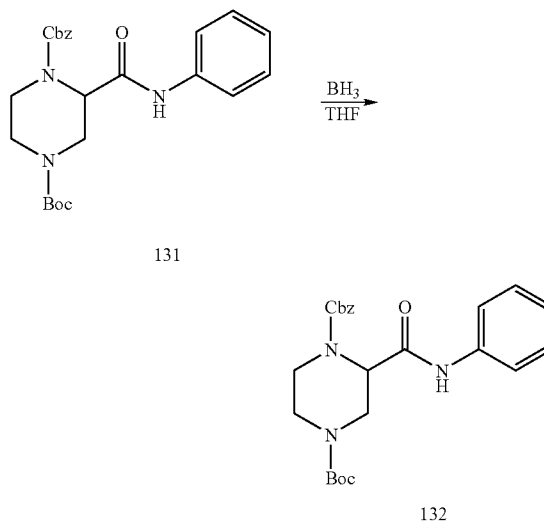
132
