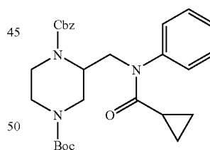
133
