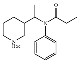
191 single enantiomer
