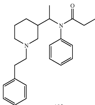
195 single enantiomer
