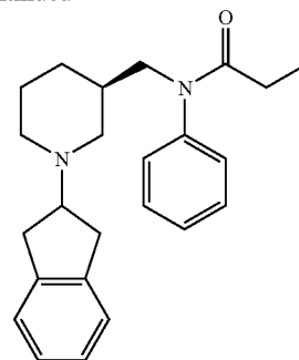
199
