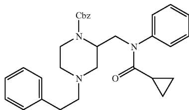
134
