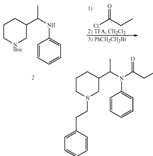
129
