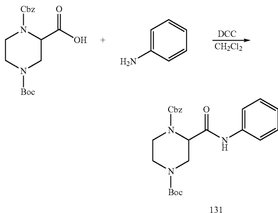
131
