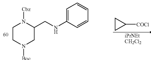
132
