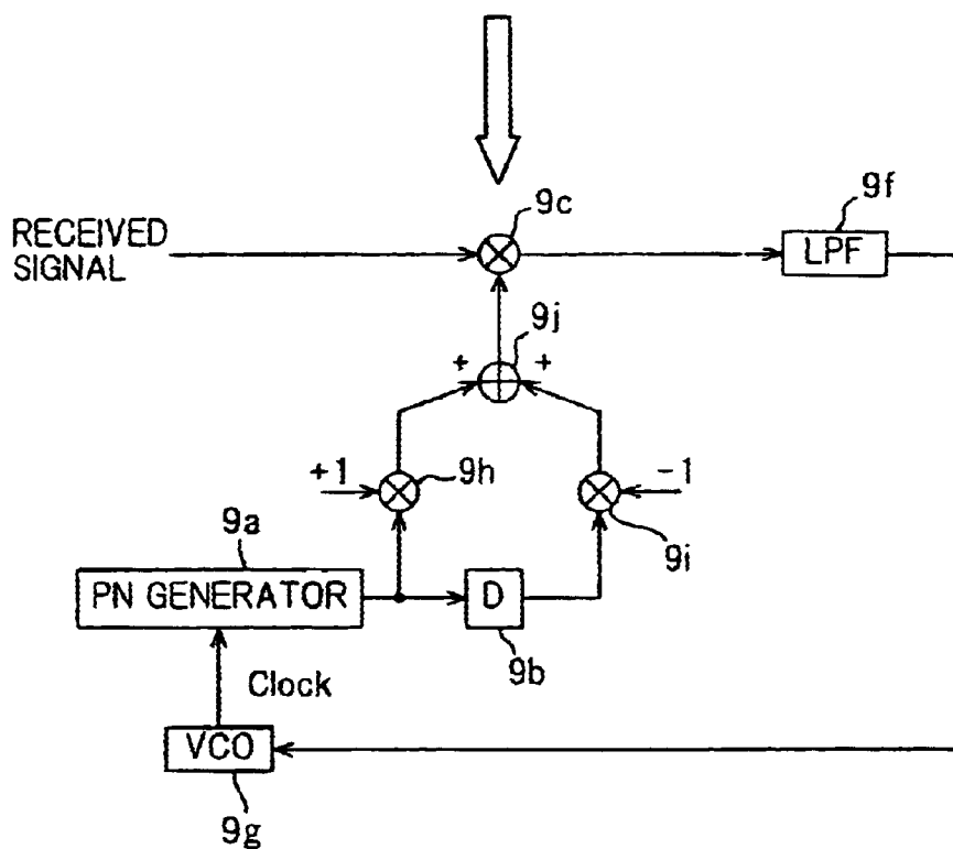
FIG. 25b (PRIOR ART)
