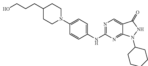
Co. No. 94; Ex. [B7]
