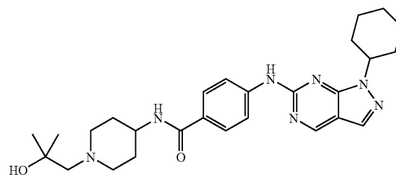
Co. No. 98; Ex. [B9]; mp. 233-236° C.
