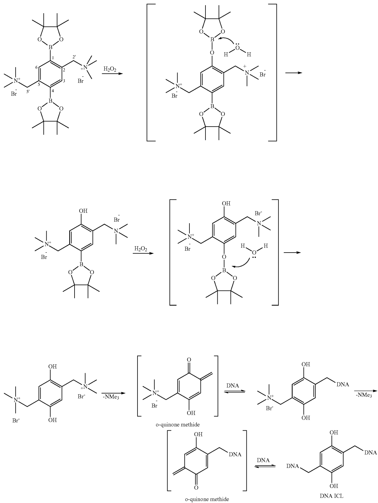
Scheme 16.
