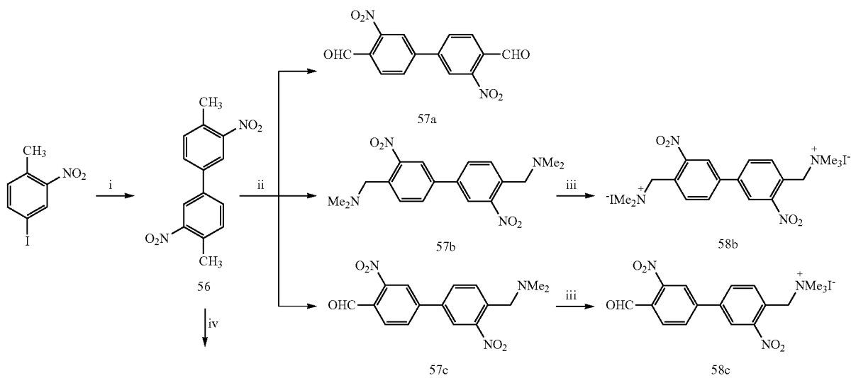
Scheme 11. Exemplary Syntheses
