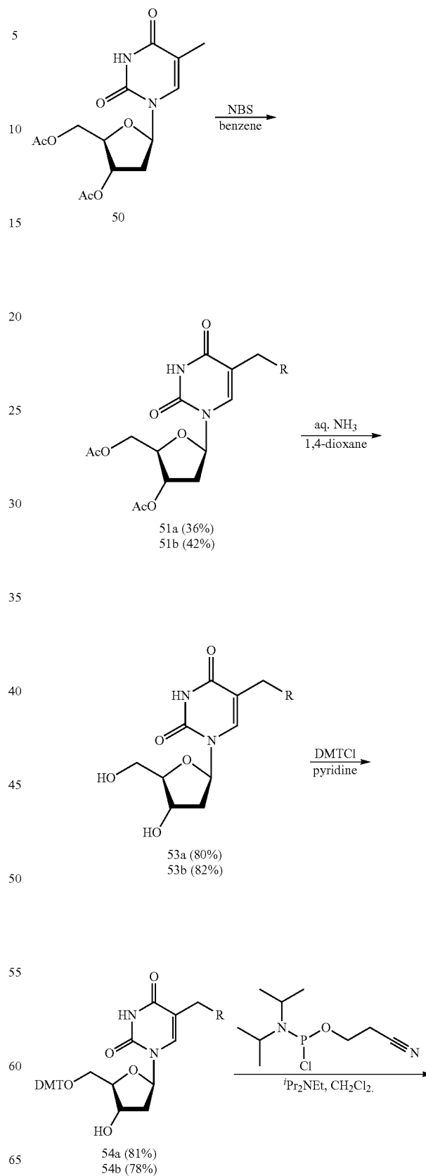
Scheme 13. Exemplary Syntheses
