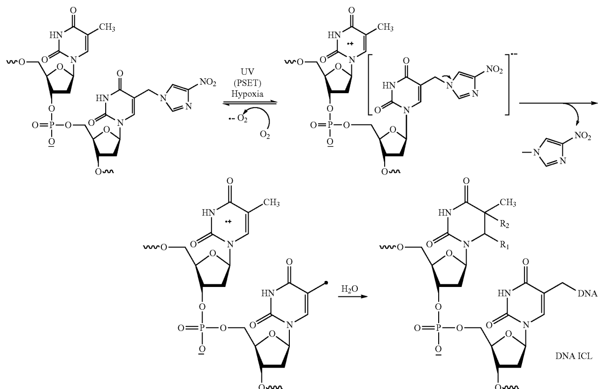
Scheme 17.
