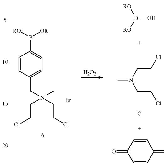
Scheme 14.
