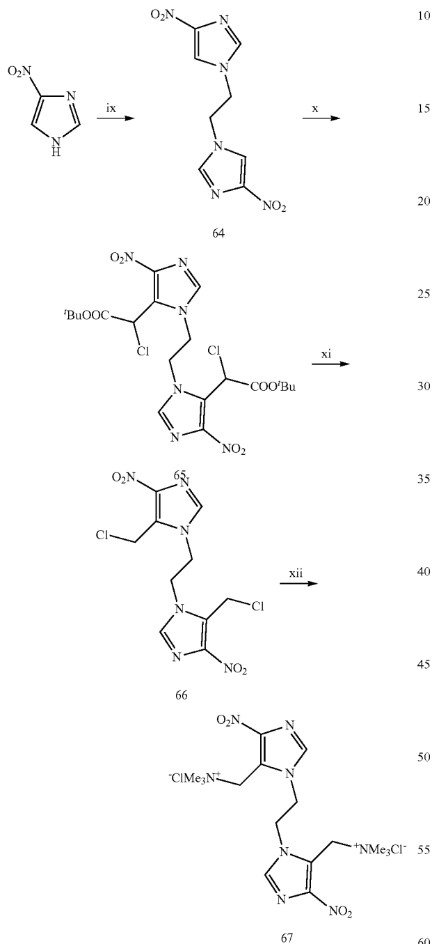
Scheme 12. Exemplary Syntheses
