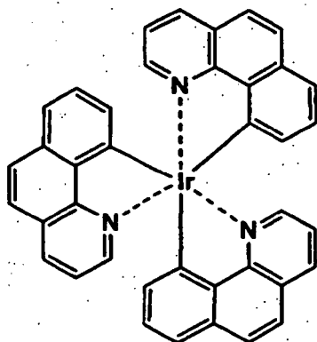
Ir-5
