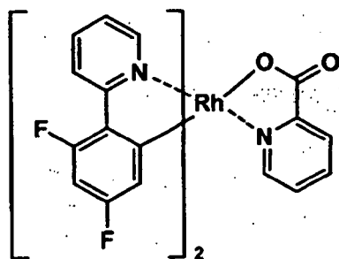
Rh-2
