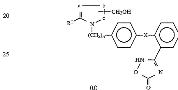
(If)
