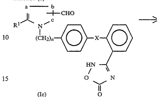
(Ie)
