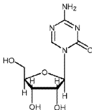
5-Azacytidine.
