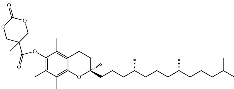
(MTC-VitE)
