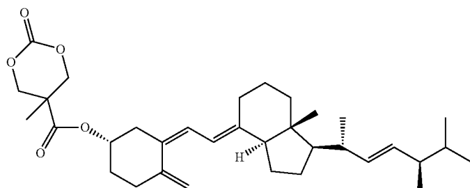
(MTC-VitD2)
