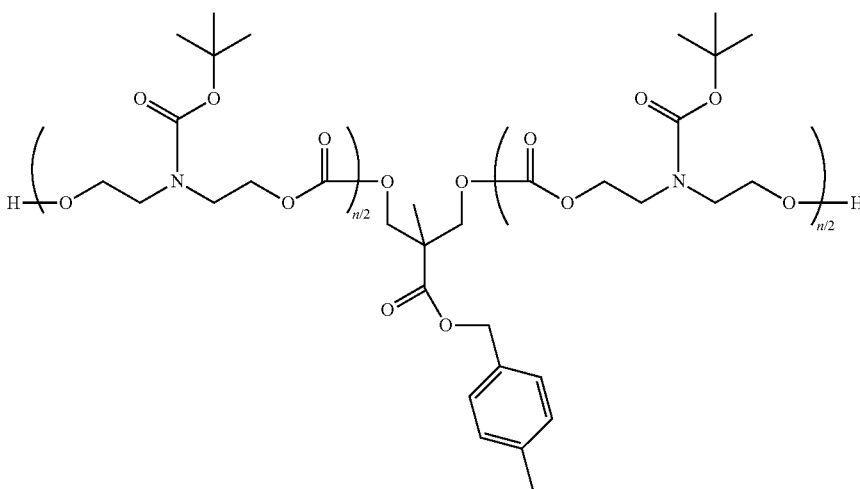
P-7 n = 50
