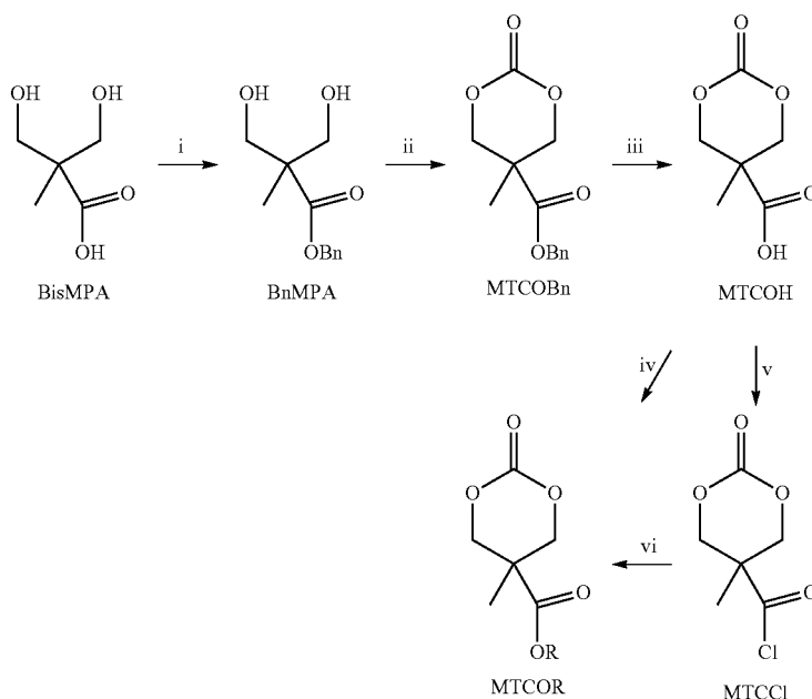
Scheme I.
