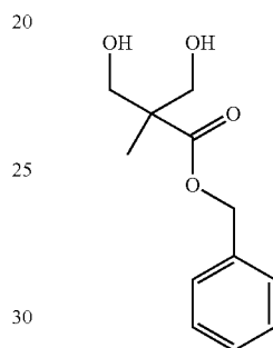
BnMPA
