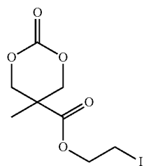
(MTC-EtI)
