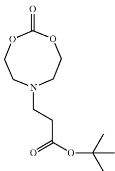
DXA-tBuP
