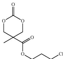
(MTC-PrCl)
