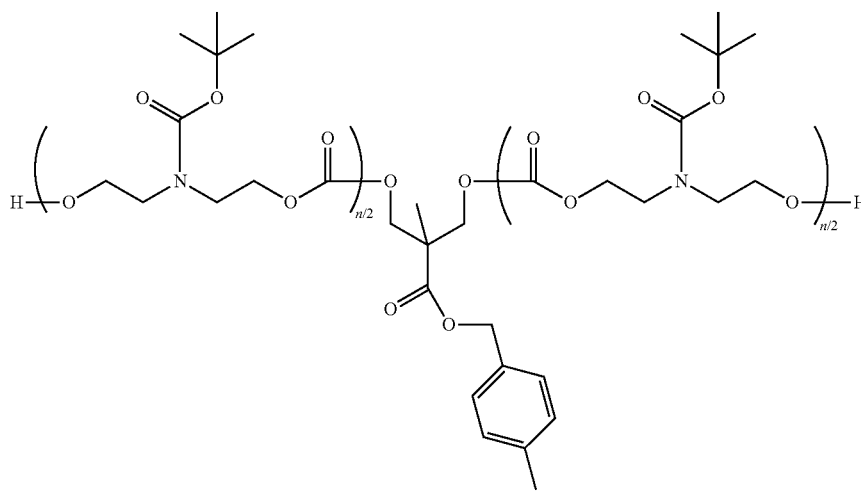
P-7 n = 50
