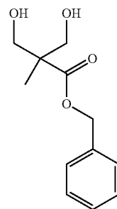
(BnMPA)
