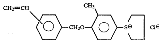
2-VBTHC
