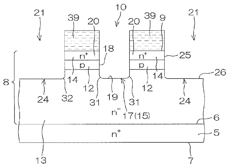
A-A SECTION
