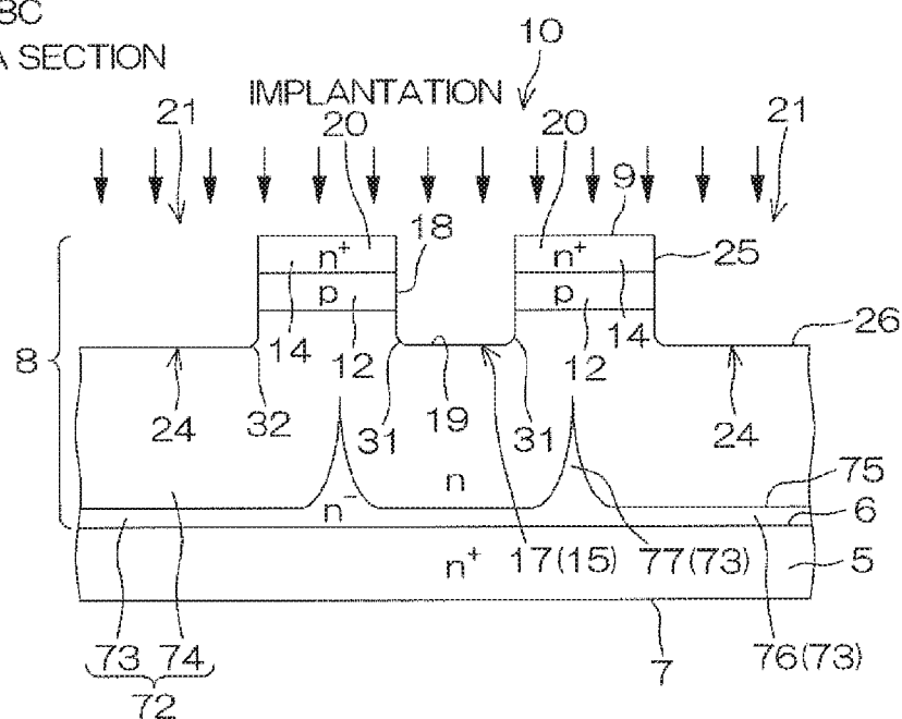
FIG. 8C
