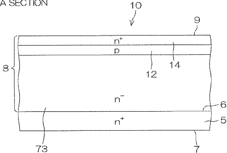
FIG. 8A A-A SECTION
