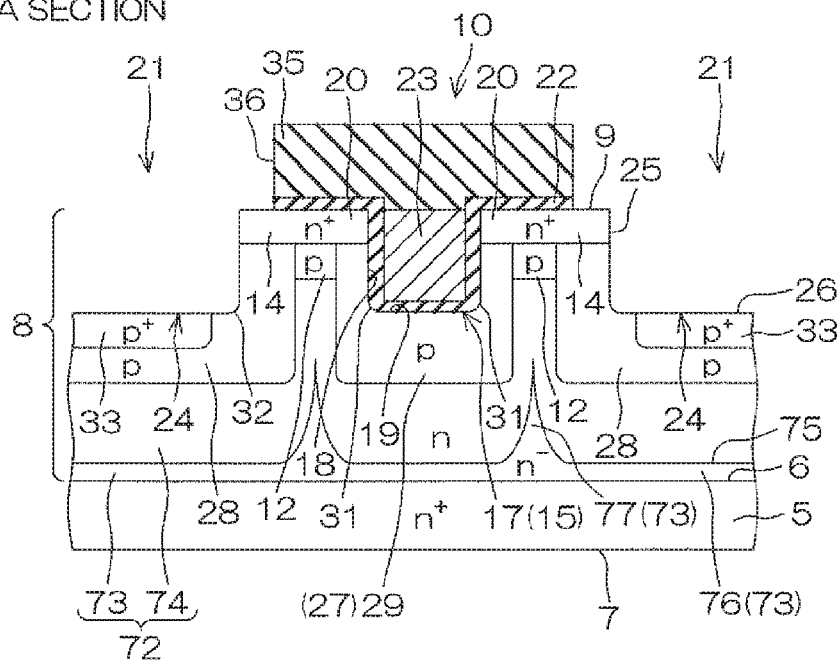
A-A SECTION
