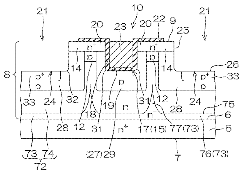
FIG. 8H A-A SECTION
