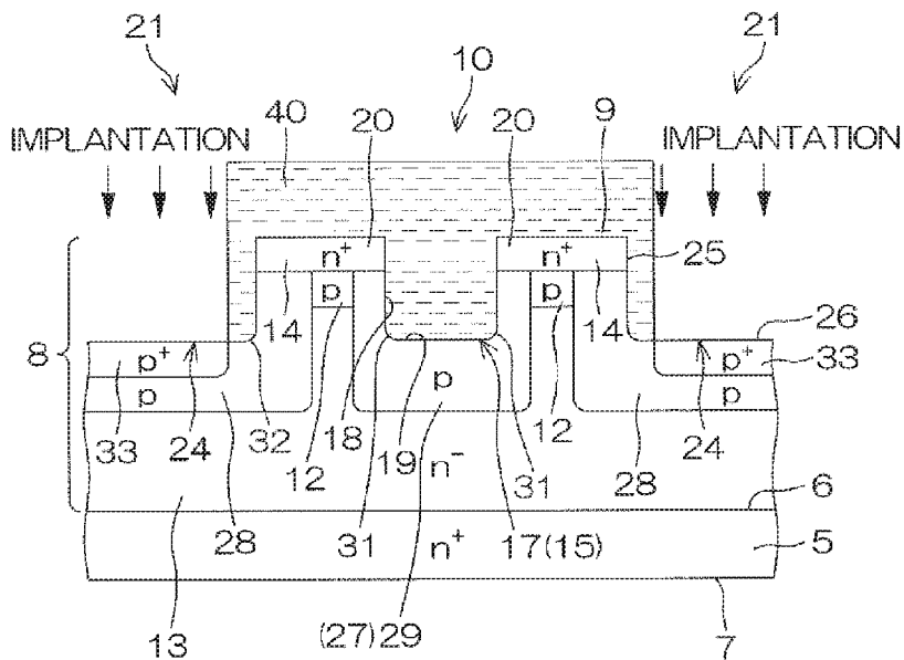
A-A SECTION
