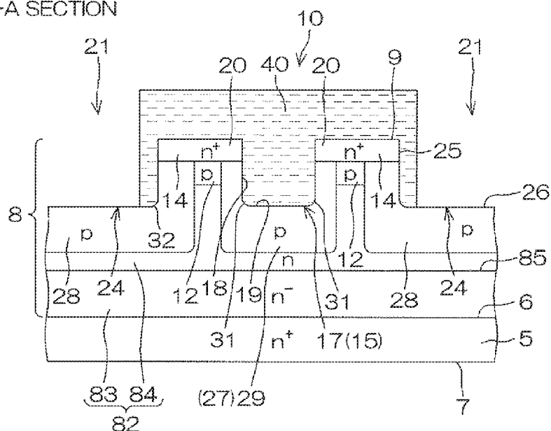
FIG. 11E A-A SECTION
