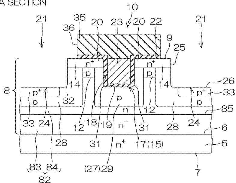
FIG. 11H A-A SECTION
