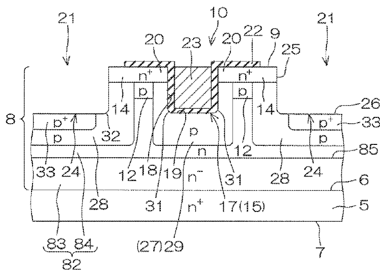
FIG. 11G A-A SECTION
