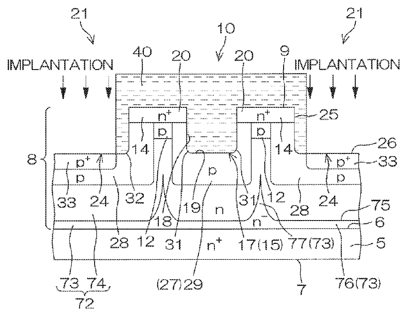
FIG. 8G
