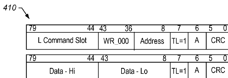
FIG. 4A
