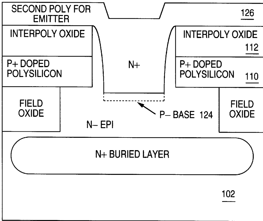
FIG. 1E (PRIOR ART)
