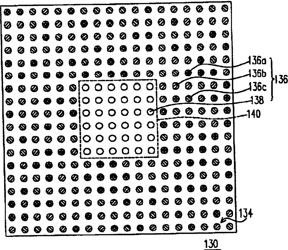
FIG. 2B(PRIOR ART)
