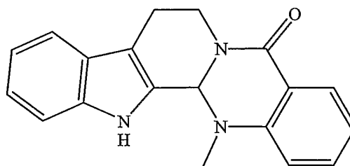
evodiamine
